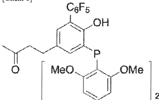
[Chem 6]
