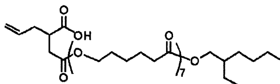
Macromonomer A5
