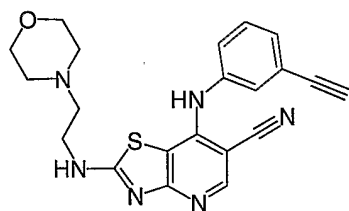
Cpd. No. 13
