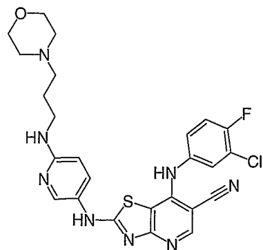
Cpd. No. 29
