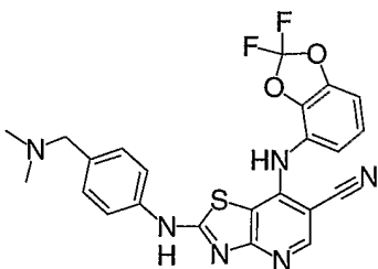
Cpd. No. 27
