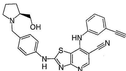
Cpd. No. 13
