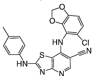
Cpd. No. 35
