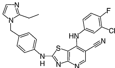
Cpd. No. 3
