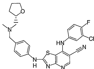
Cpd. No. 17
