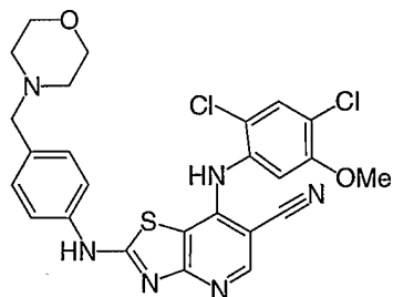
Cpd. No. 49
