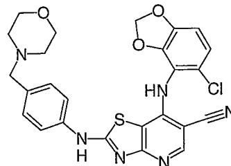
Cpd. No. 20
