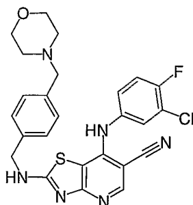
Cpd. No. 24
