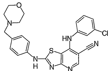
Cpd. No. 19
