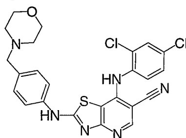
Cpd. No. 36
