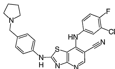
Cpd. No. 19
