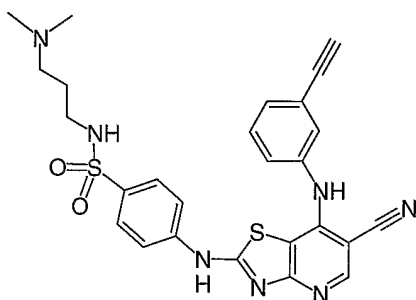
Cpd. No. 23
