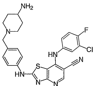
Cpd. No. 33
