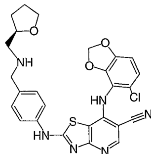
Cpd. No. 46
