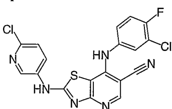
Cpd. No. 30
