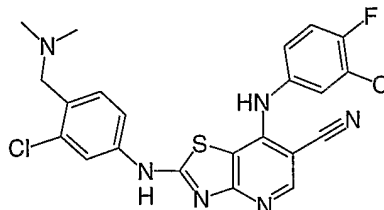
Cpd. No. 18
