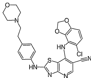
Cpd. No. 49
