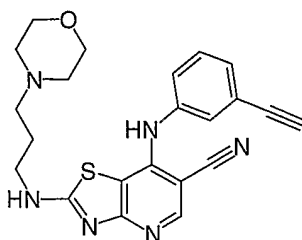
Cpd. No. 9
