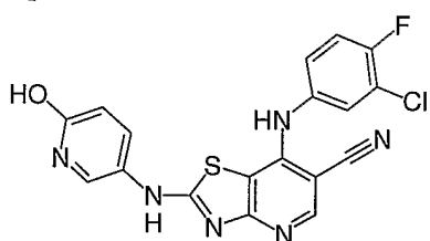
Cpd. No. 29
