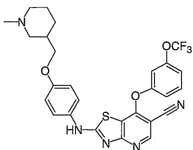
Cpd. No. 39
