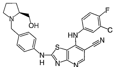
Cpd. No. 6
