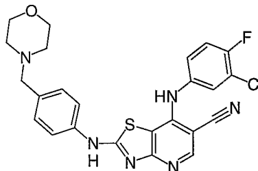
Cpd. No. 4
