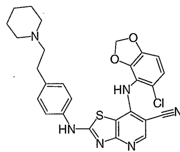
Cpd. No. 50
