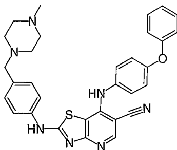
Cpd. No. 51
