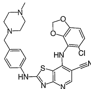
Cpd. No. 48
