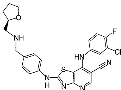
Cpd. No. 23
