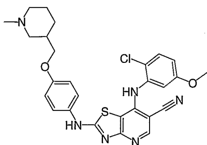
Cpd. No. 37
