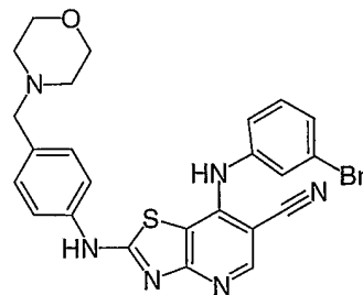
Cpd. No. 50
