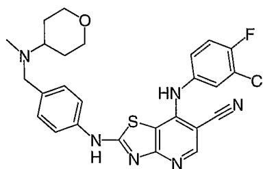
Cpd. No. 16
