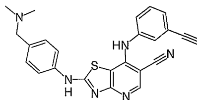
Cpd. No. 10
