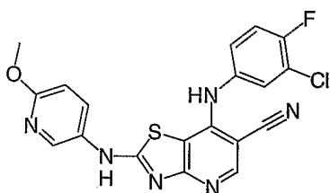
Cpd. No. 26
