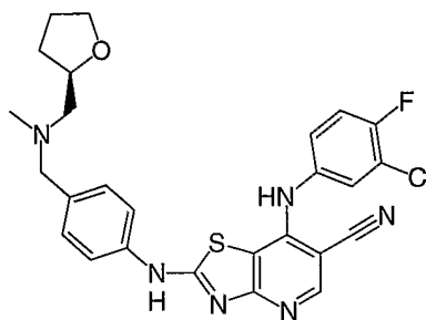
Cpd. No. 16
