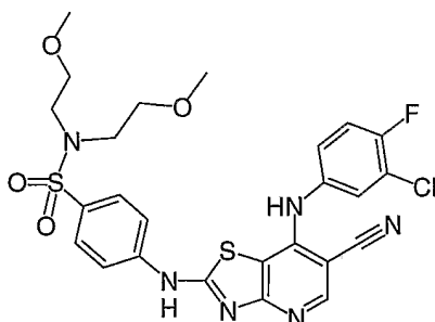
Cpd. No. 7
