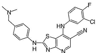
Cpd. No. 3
