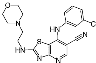
Cpd. No. 12
