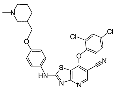
Cpd. No. 38
