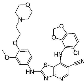
Cpd. No. 44
