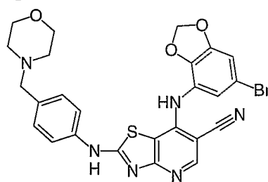
Cpd. No. 32
