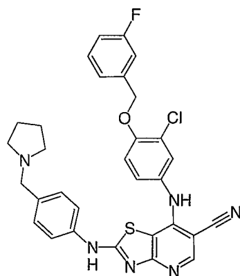
Cpd. No. 26
