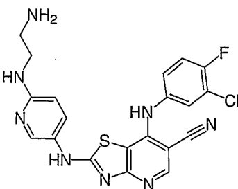
Cpd. No. 30
