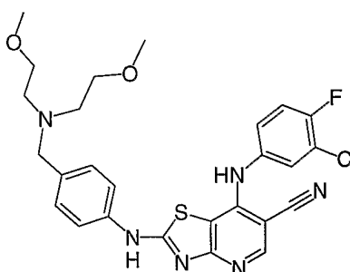
Cpd. No. 6
