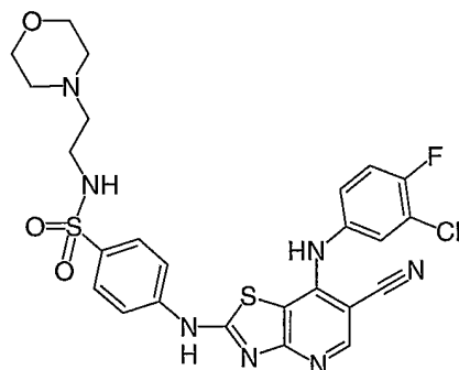
Cpd. No. 9
