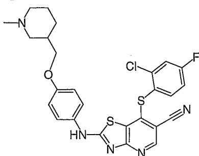
Cpd. No. 39
