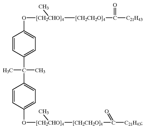
di-(PEG-4, PPG-4) Bisphenol A dibehenate
