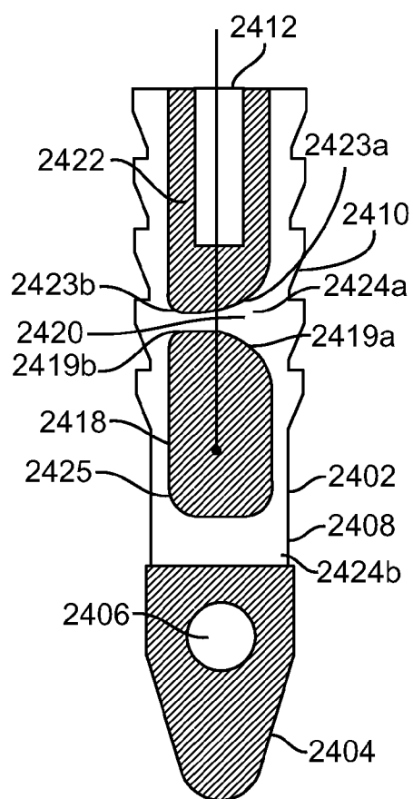
VIEW A-A
