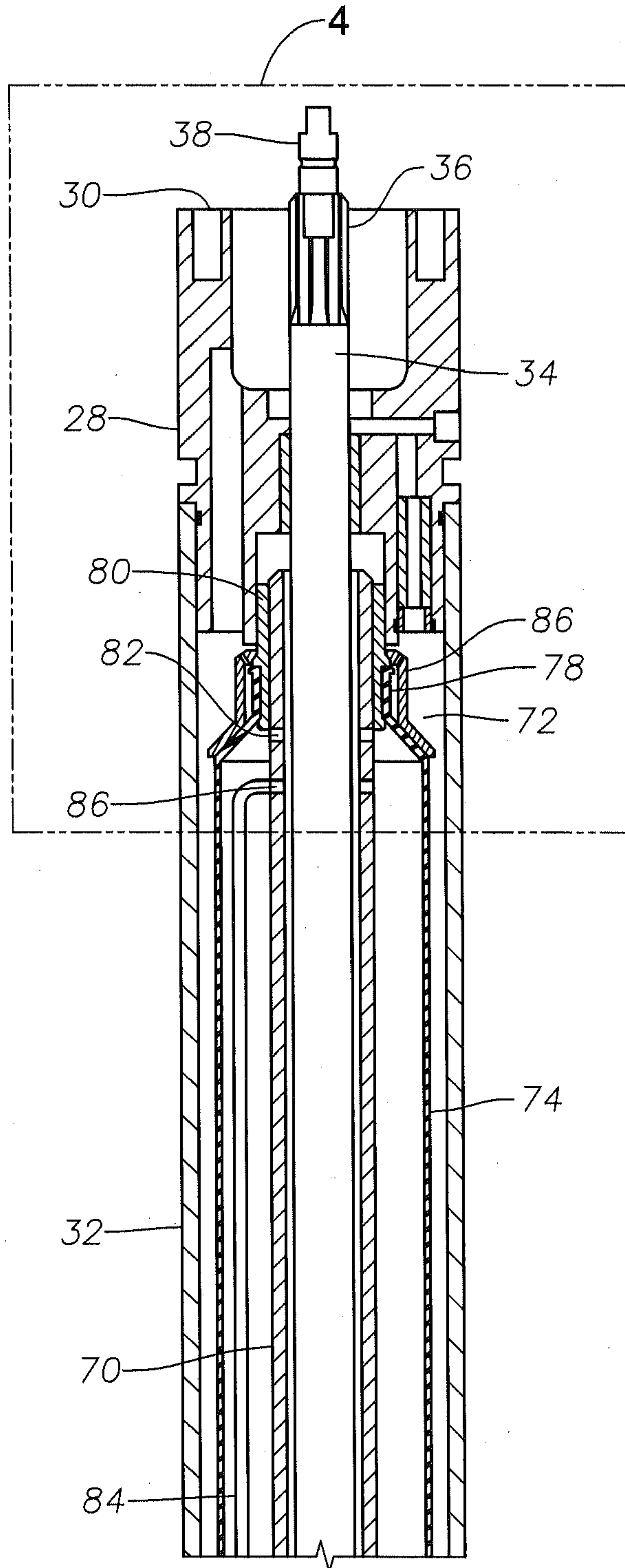
FIG. 2A
