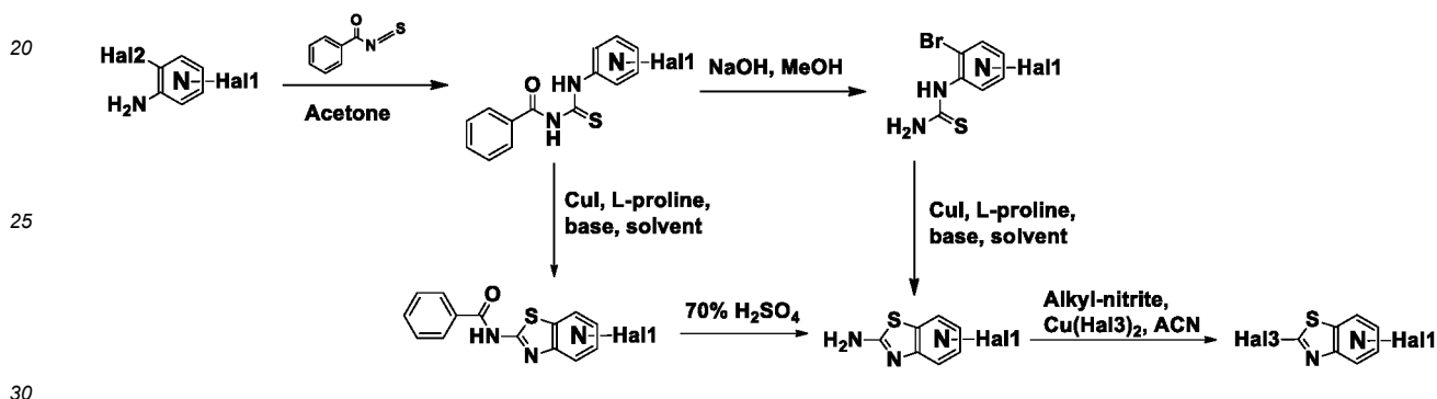
Scheme 1a
