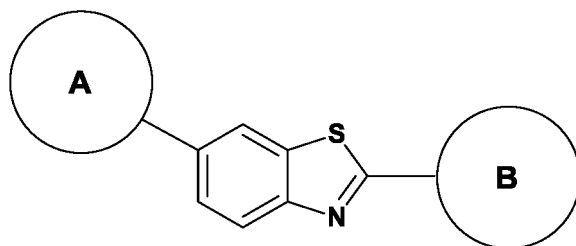
(Ig)
