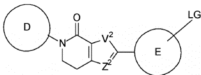
(IVb)
