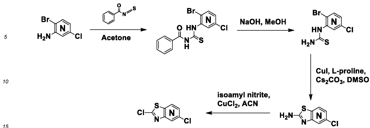
Scheme 1a
