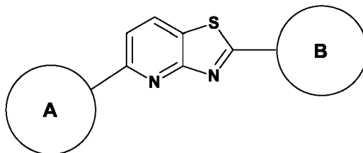
(Ih)
