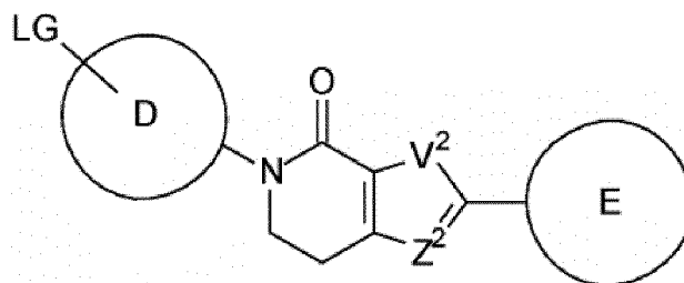
(IVa)
