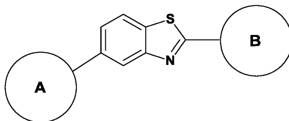
(If)
