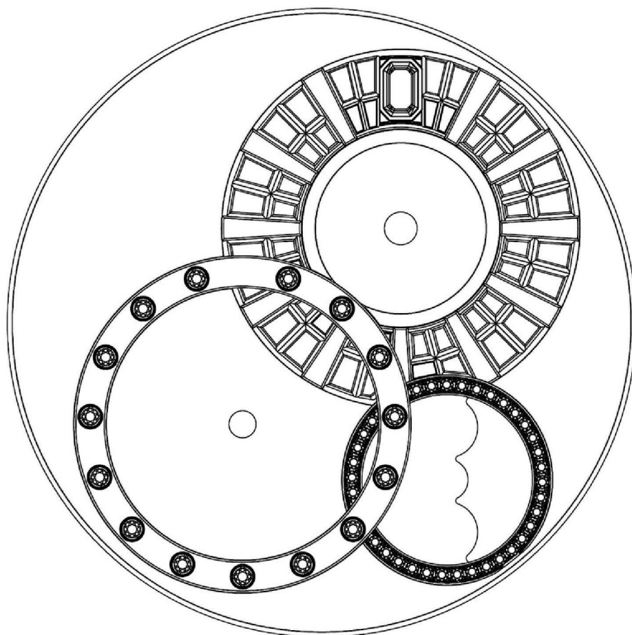
【前視圖】
