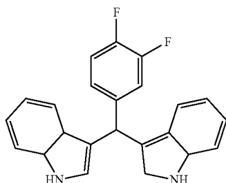
DIM-DF (HN18)
