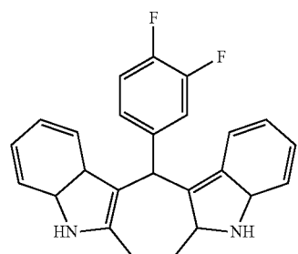
MeDIM-DF (HN34)
