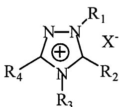
Triazolium
