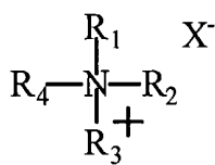
Ammonium
