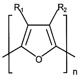
Polyfuran
