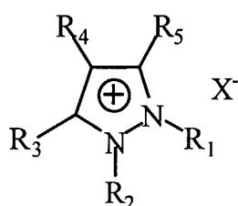
Pyrazolium
