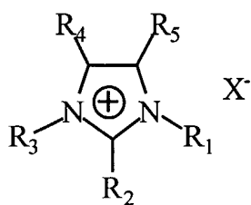
Imidazolium
