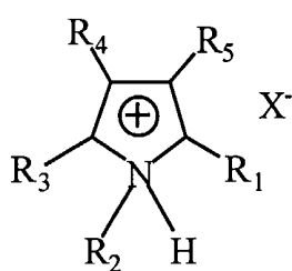
Pyrrolium
