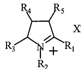
Pyrrolinium
