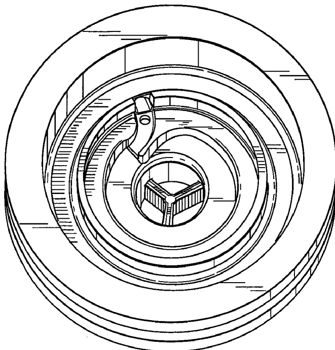
FIG. 25b
