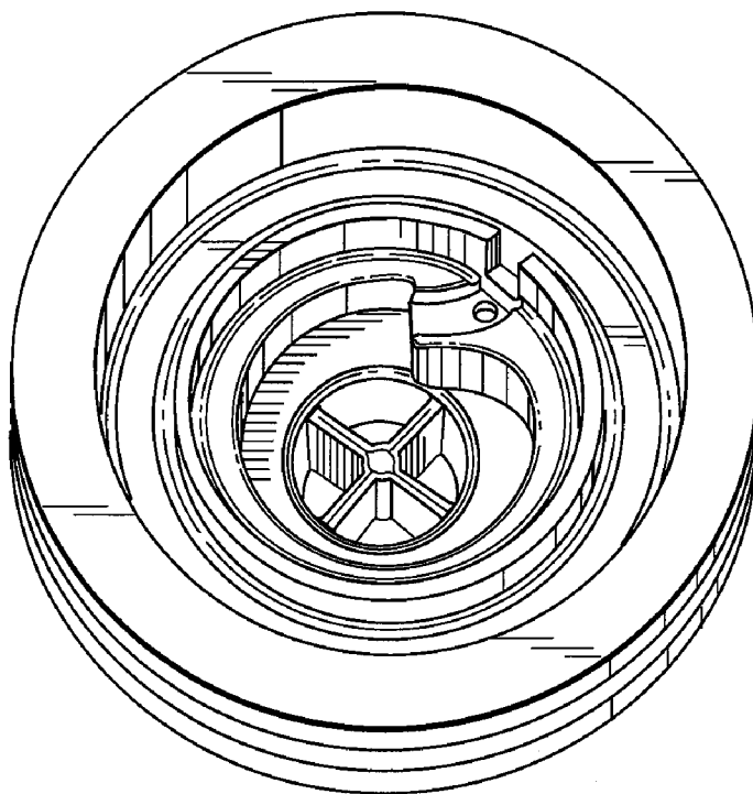
FIG. 25d
