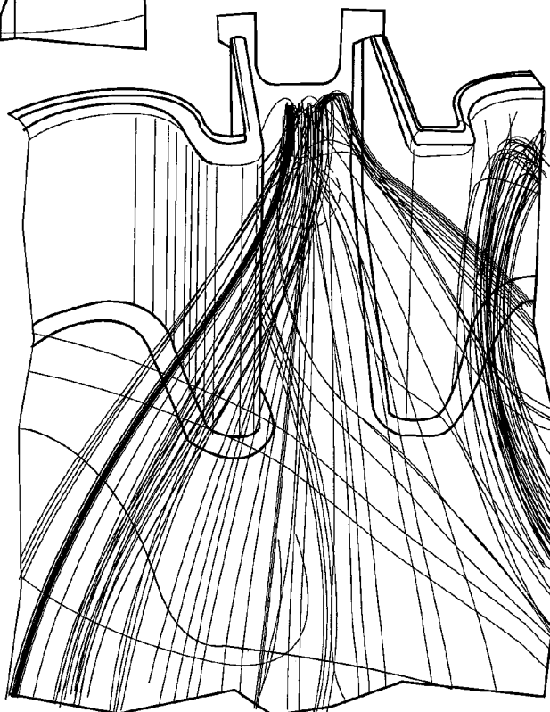
FIG. 12b
