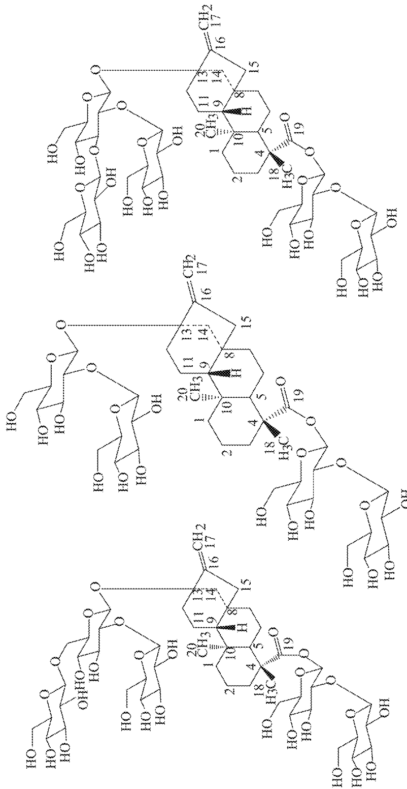
Rebaudioside D
