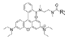
rhodamineB -DMEDA linker
