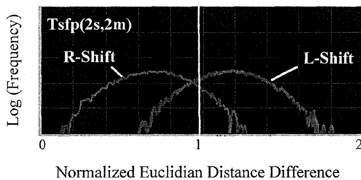
(b) Tsfp(2s,2m) Edge Shift = +0.2T
