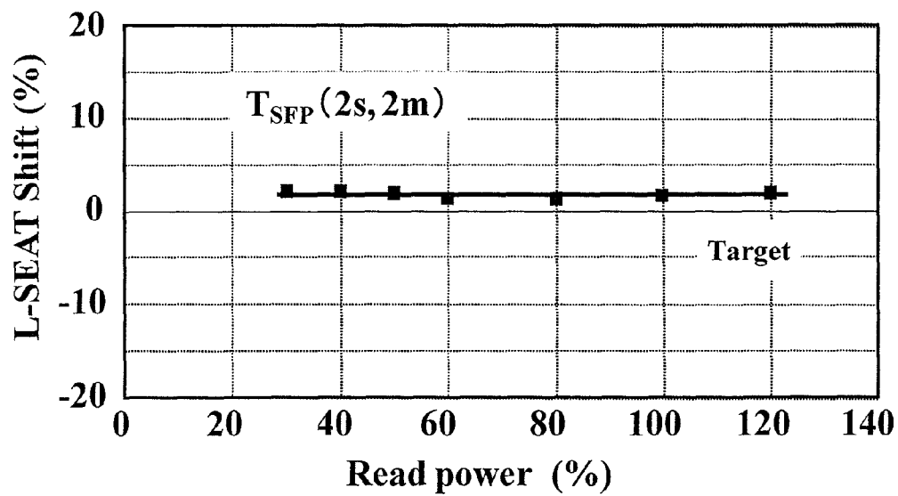
(b) Edge Shift
