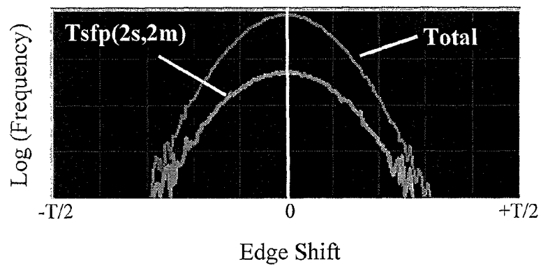
(a) Tsfp(2s,2m) Edge Shift = 0.0T
