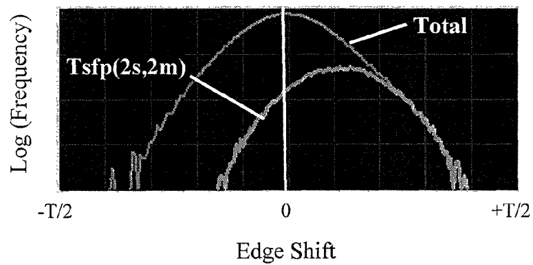
(b) Tsfp(2s,2m) Edge Shift = +0.2T
