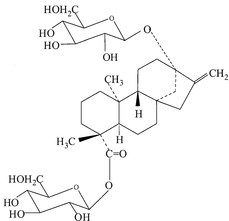
Rubusoside
