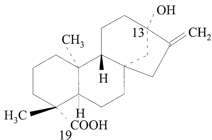
Steviol
