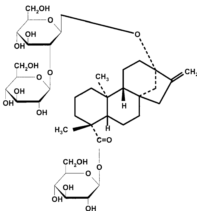
Stevioside
