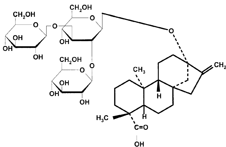
Rebaudioside B
