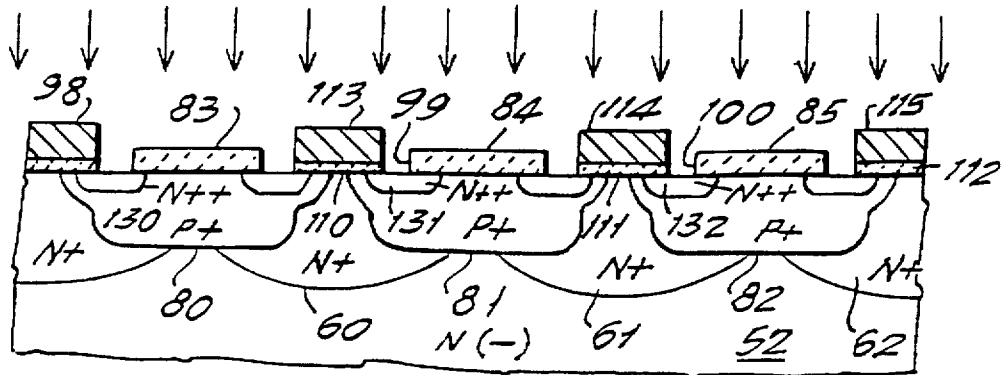
FIG. 17. ARSENIC
