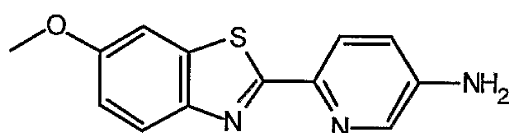
6-(6-methoxy-1,3-benzothiazol-2-yl)pyridin-3-amine
