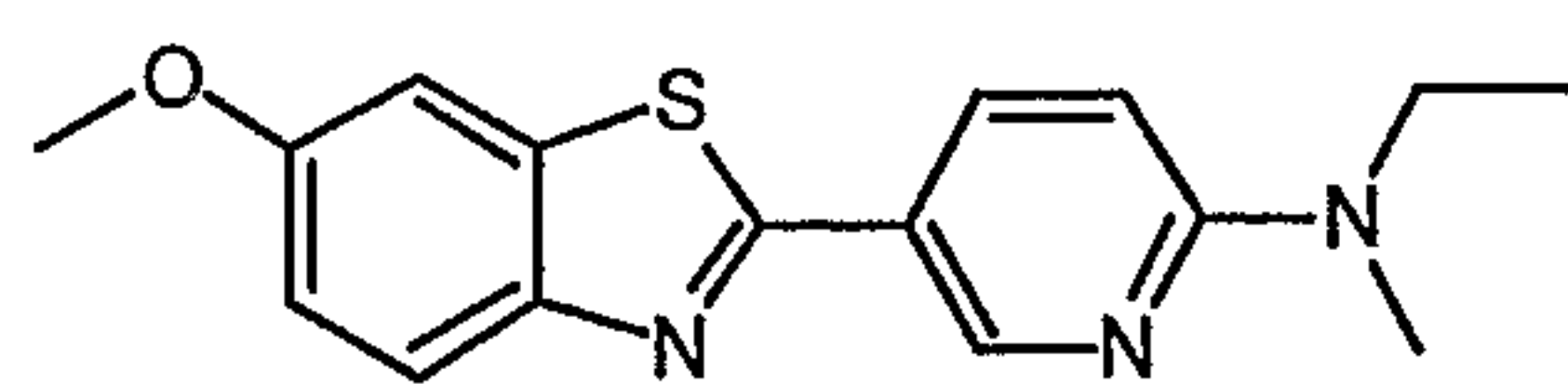
N-ethyl-5-(6-methoxy-1,3-benzothiazol-2-yl)-N-methylpyridin-2-amine
