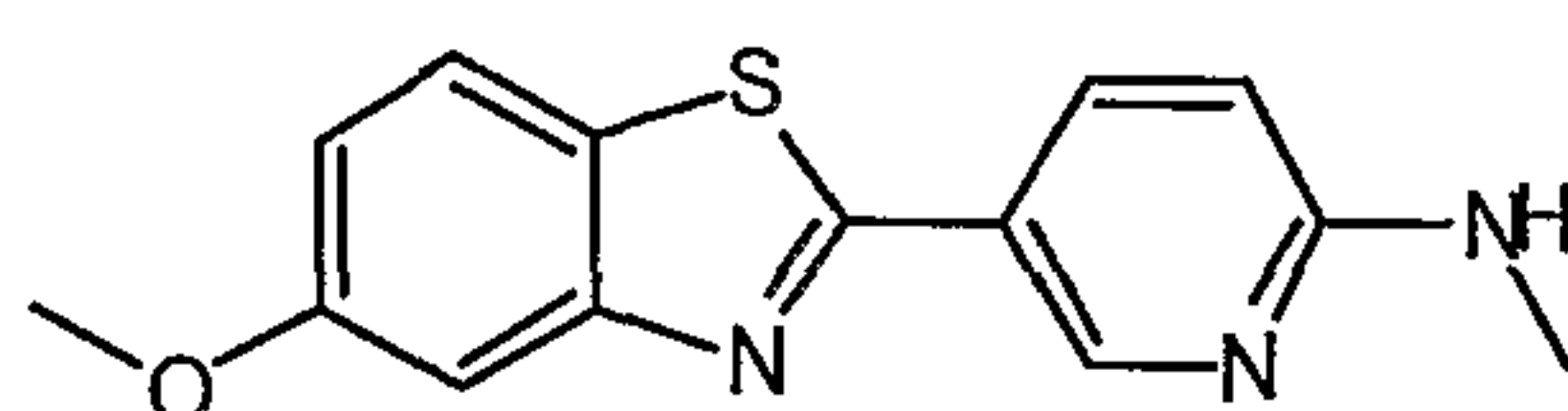
5-(5-methoxy-1,3-benzothiazol-2-yl)-N-methylpyridin-2-amine
