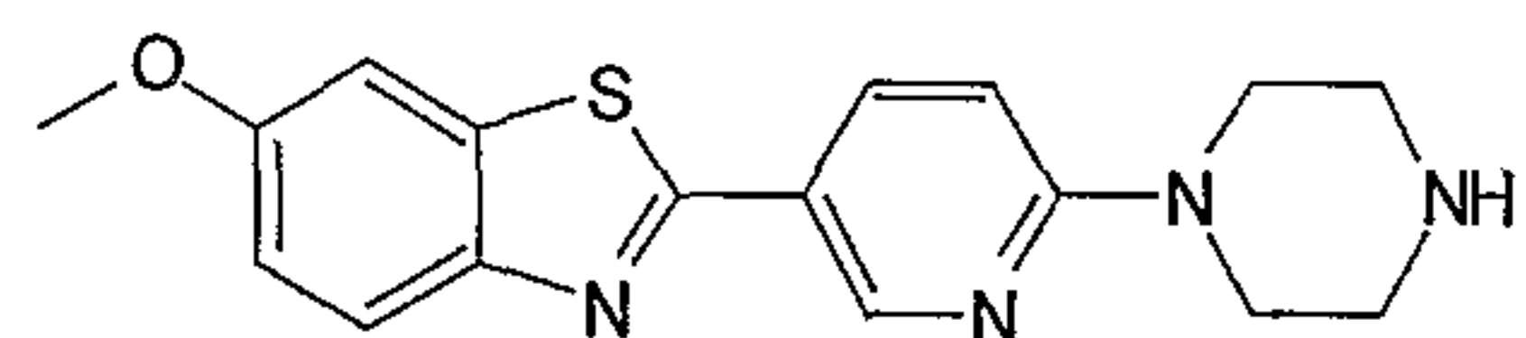
6-methoxy-2-(6-piperazin-1-ylpyridin-3-yl)-1,3-benzothiazole
