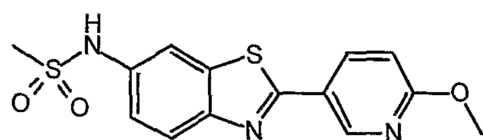
N-[2-(6-Methoxypyridin-3-yl)-1,3-benzothiazol-6-yl]methanesulfonamide
