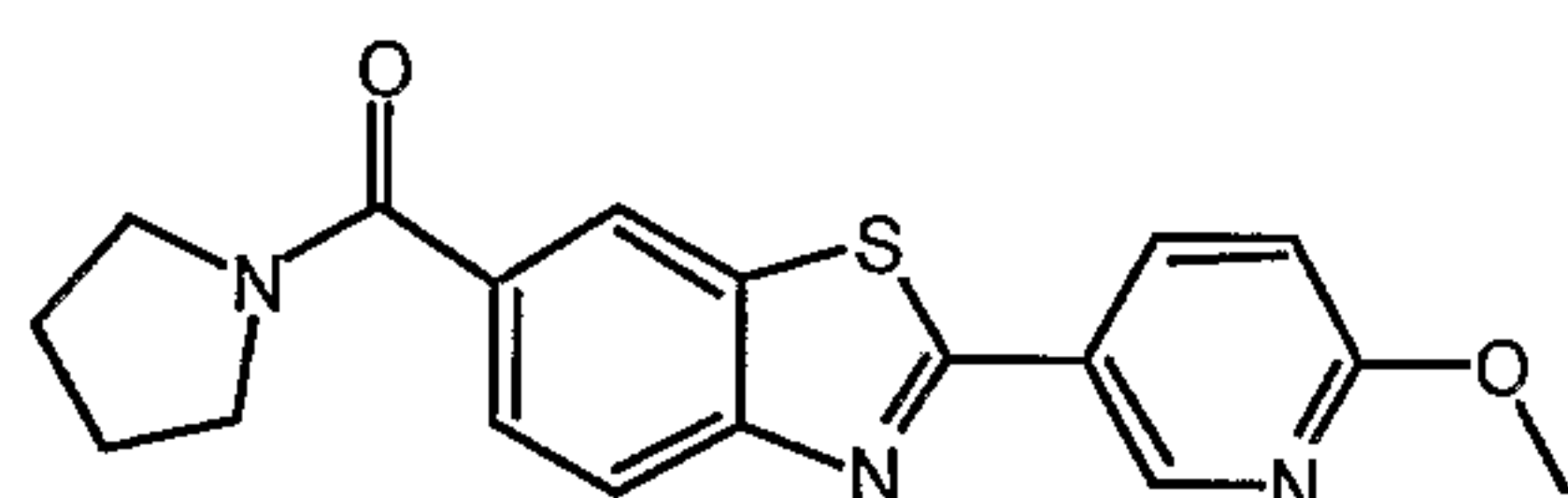
2-(6-Methoxypyridin-3-yl)-6-(pyrrolidin-1-ylcarbonyl)-1,3-benzothiazole
