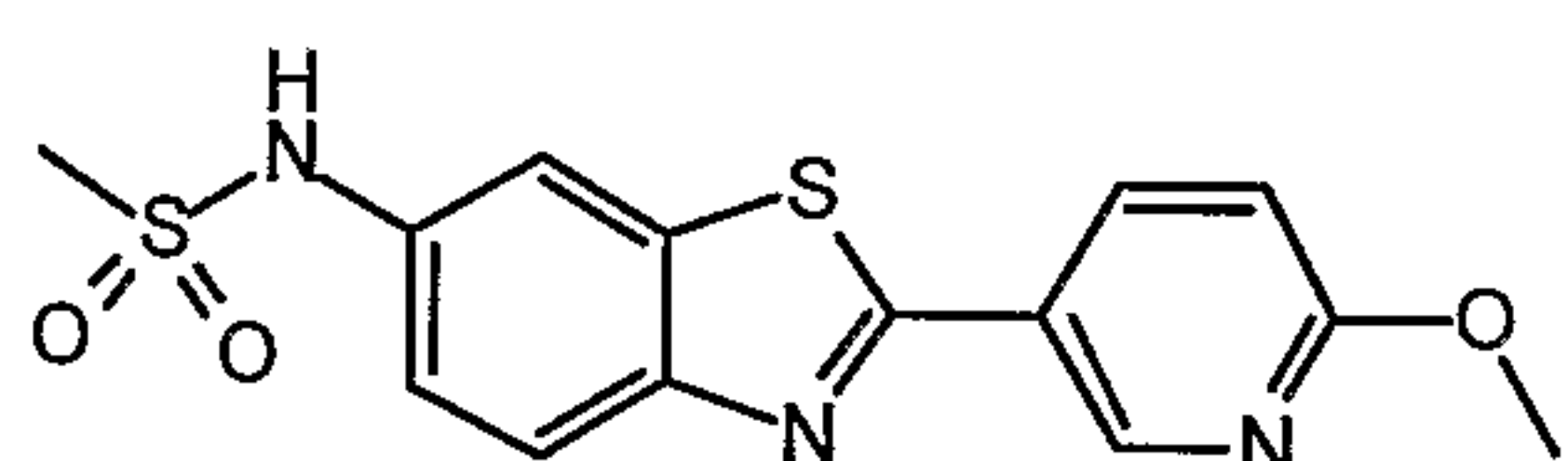
N-[2-(6-Methoxypyridin-3-yl)-1,3-benzothiazol-6-yl]methanesulfonamide
