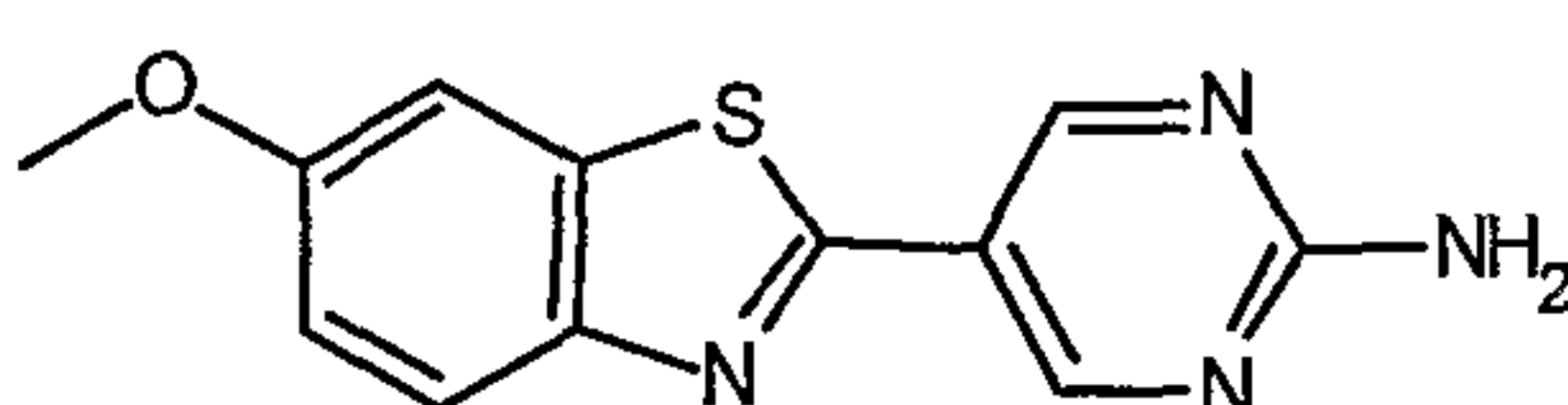
5-(6-methoxy-1,3-benzothiazol-2-yl)pyrimidin-2-amine
