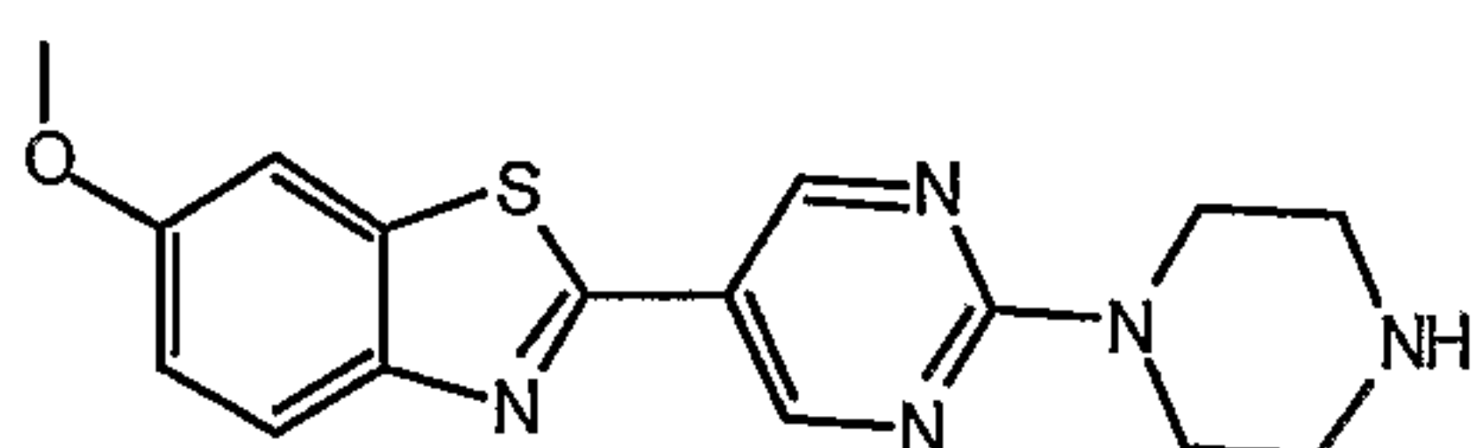
6-methoxy-2-(2-piperazin-1-yl)pyrimidin-5-yl)-1,3-benzothiazole
