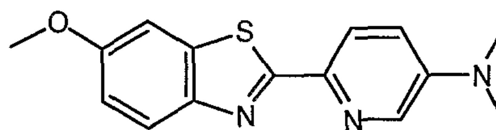
6-(6-methoxy-1,3-benzothiazol-2-yl)-N,N-dimethylpyridin-3-amine
