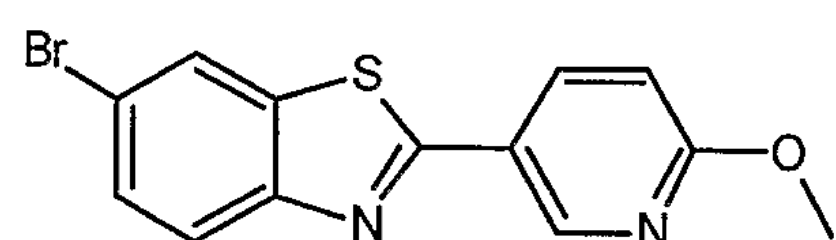
6-Bromo-2-(6-methoxypyridin-3-yl)-1,3-benzothiazole
