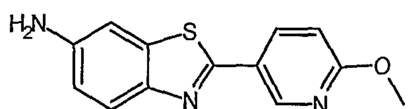
2-(6-Methoxypyridin-3-yl)-1,3-benzothiazol-6-amine
