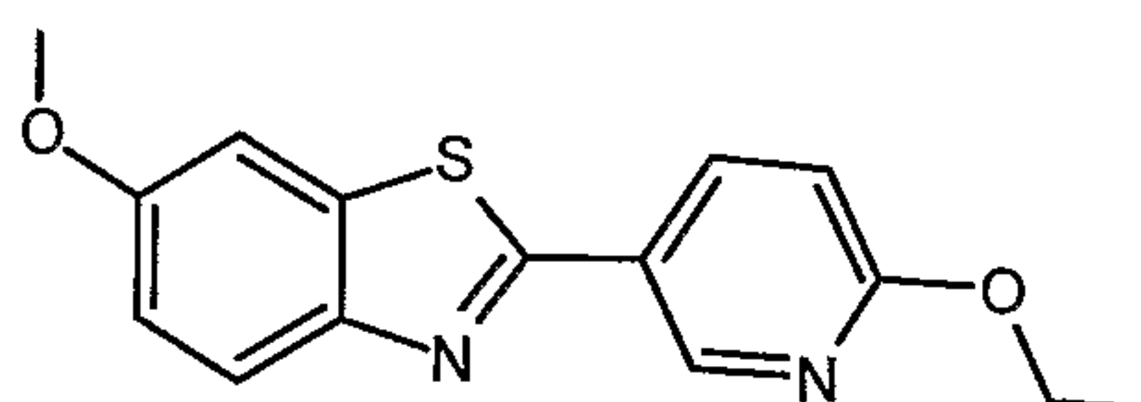
2-(6-ethoxypyridin-3-yl)-6-methoxy-1,3-benzothiazole
