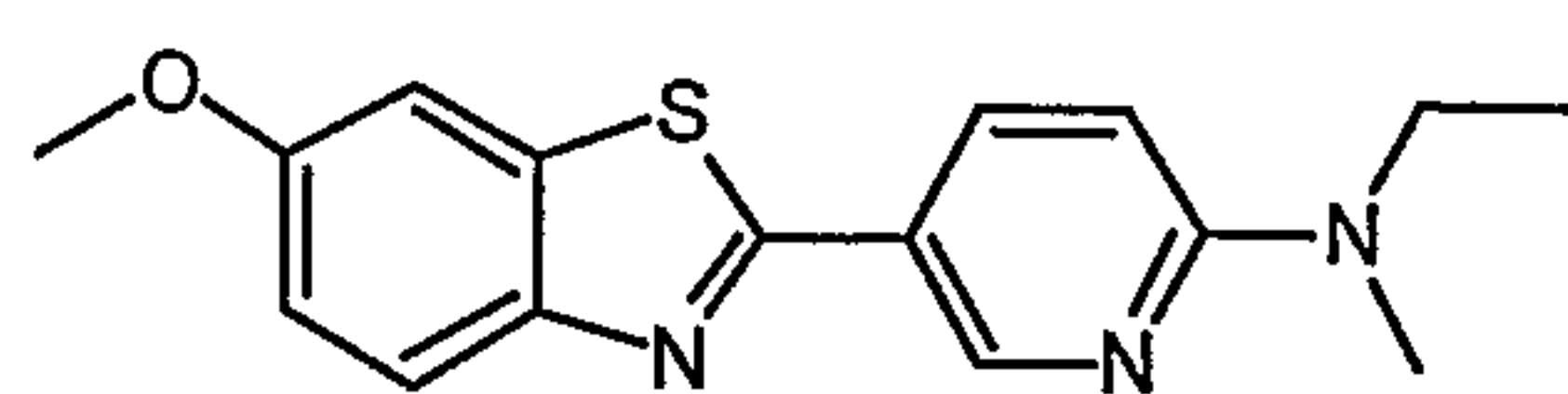
N-ethyl-5-(6-methoxy-1,3-benzothiazol-2-yl)-N-methylpyridin-2-amine
