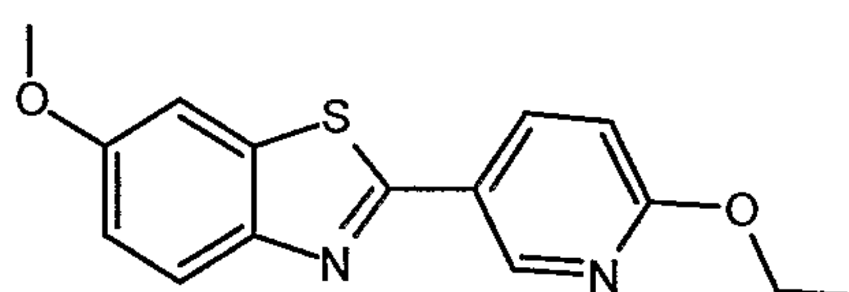
2-(6-ethoxypyridin-3-yl)-6-methoxy-1,3-benzothiazole
