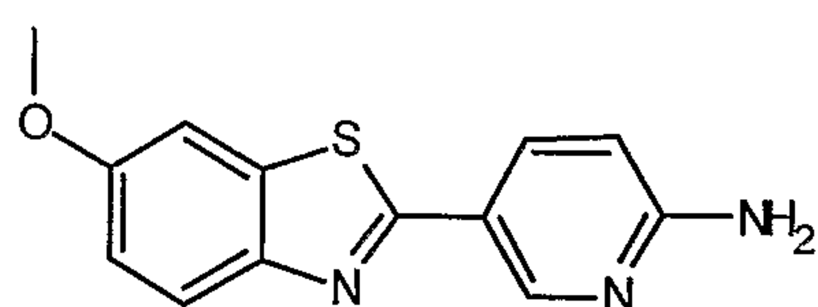
5-(6-Methoxy-1,3-benzothiazol-2-yl)pyridin-2-amine
