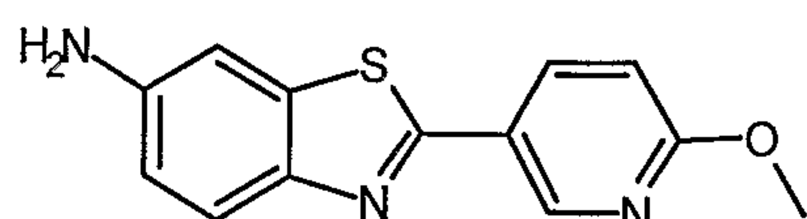
2-(6-Methoxypyridin-3-yl)-1,3-benzothiazol-6-amine
