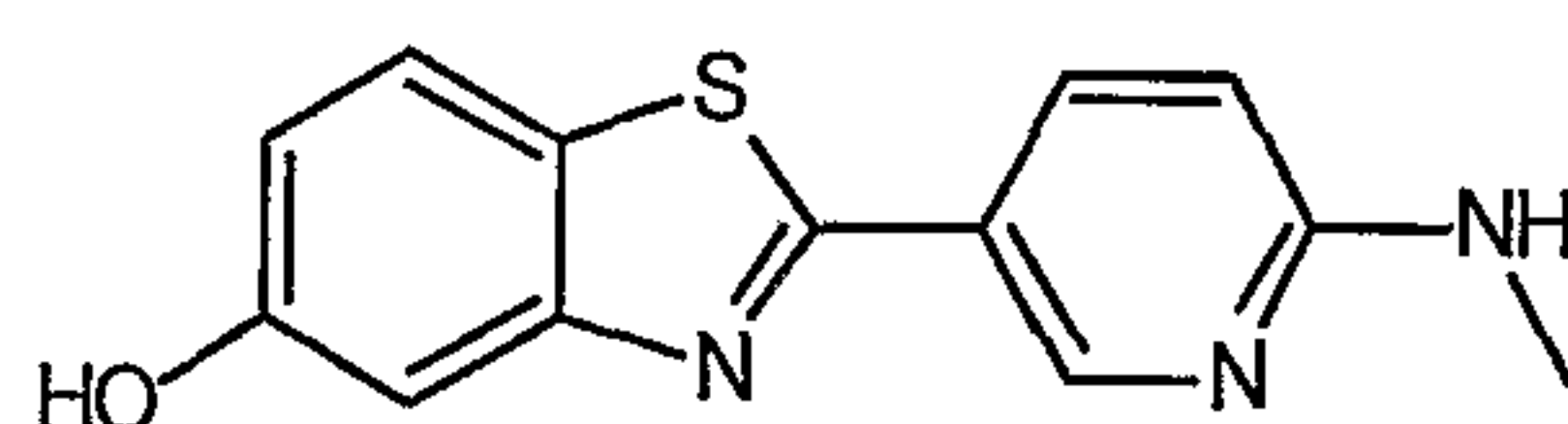
2-[6-(methylamino)pyridin-3-yl]-1,3-benzothiazol-5-ol
