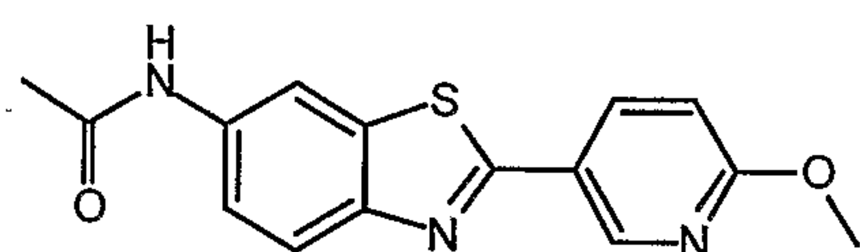
N-[2-(6-Methoxypyridin-3-yl)-1,3-benzothiazol-6-yl]acetamide
