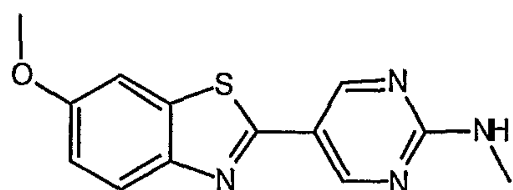
5-(6-methoxy-1,3-benzothiazol-2-yl)-N-methylpyrimidin-2-amine
