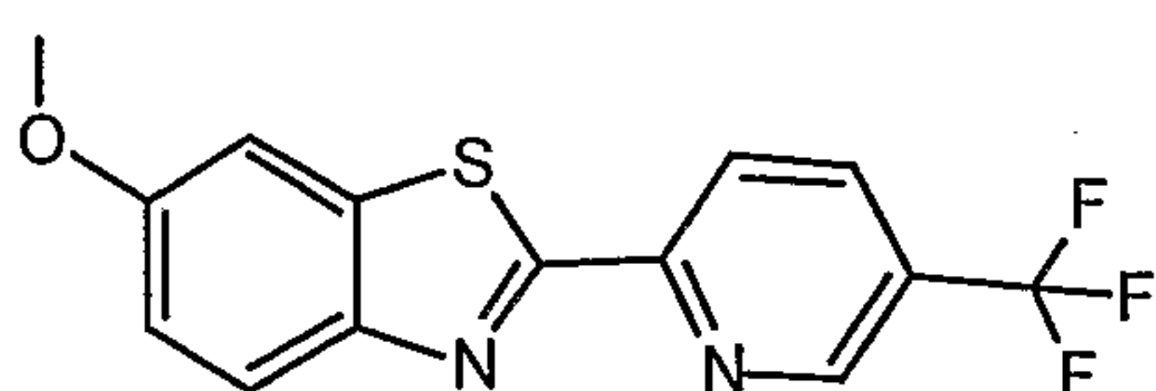
6-methoxy-2-[5-(trifluoromethyl)pyridin-2-yl]-1,3-benzothiazole
