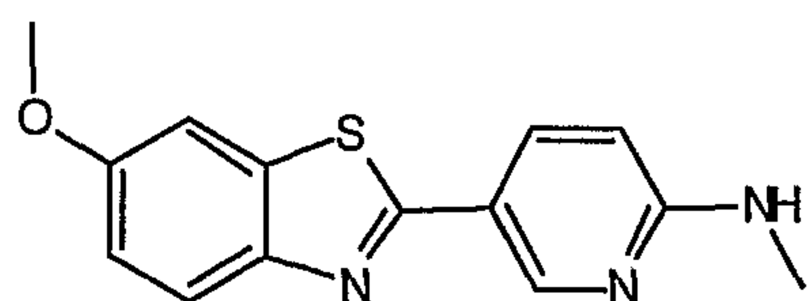
5-(6-Methoxy-1,3-benzothiazol-2-yl)-N-methylpyridin-2-amine
