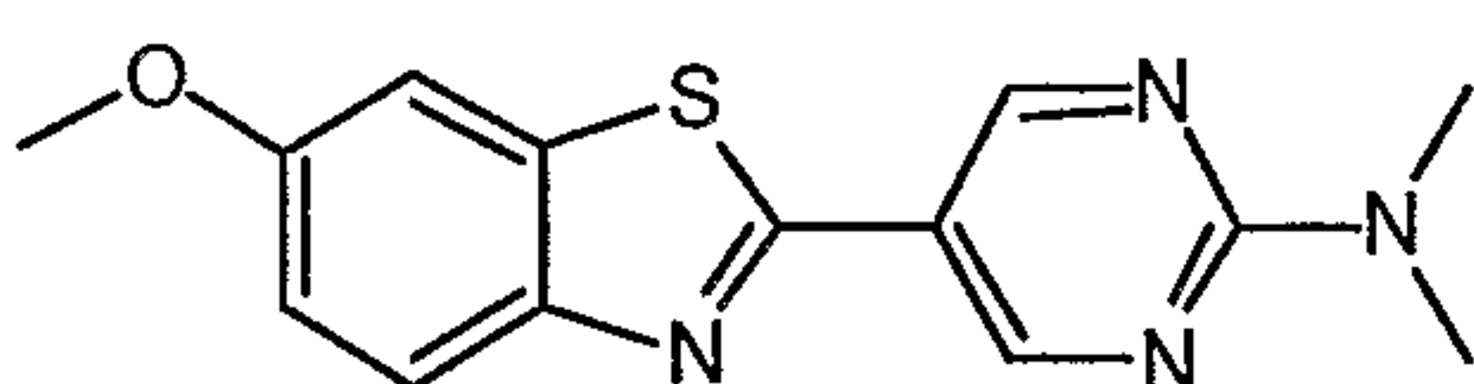
5-(6-methoxy-1,3-benzothiazol-2-yl)-N,N-dimethylpyrimidin-2-amine
