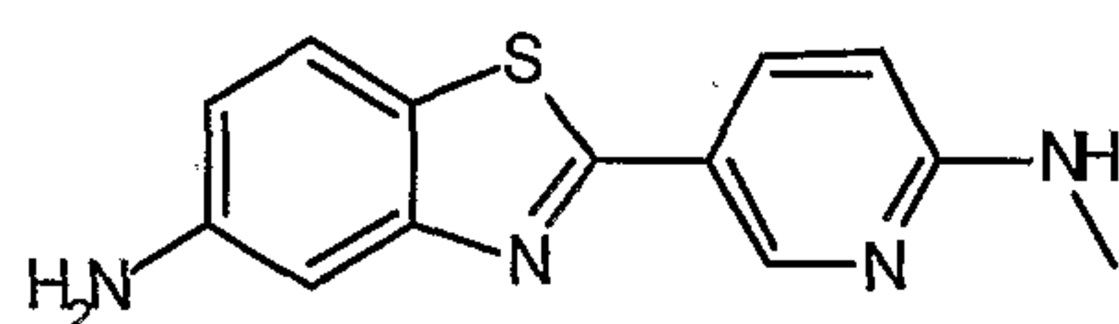
2-[6-(methylamino)pyridin-3-yl]-1,3-benzothiazol-5-amine
