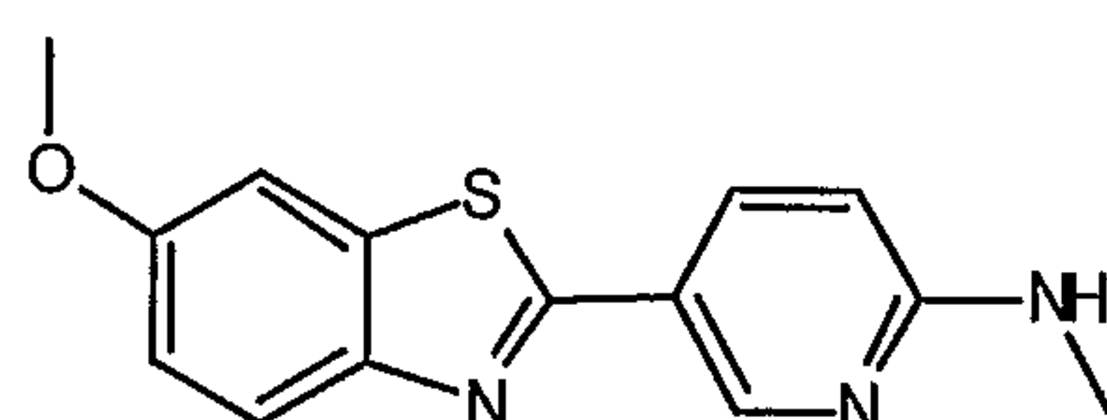
5-(6-Methoxy-1,3-benzothiazol-2-yl)-N-methylpyridin-2-amine
