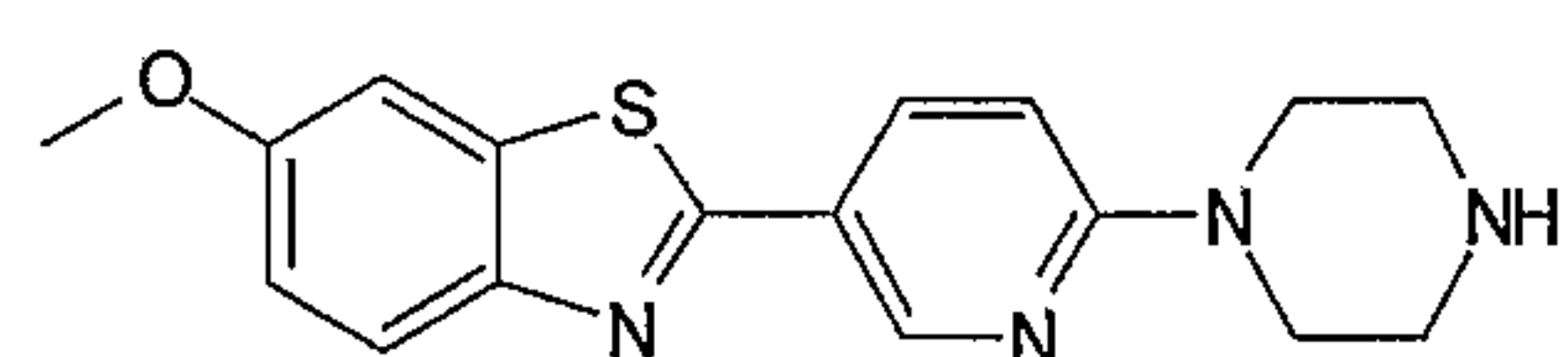
6-Methoxy-2-(6-piperazin-1-ylpyridin-3-yl)-1,3-benzothiazole
