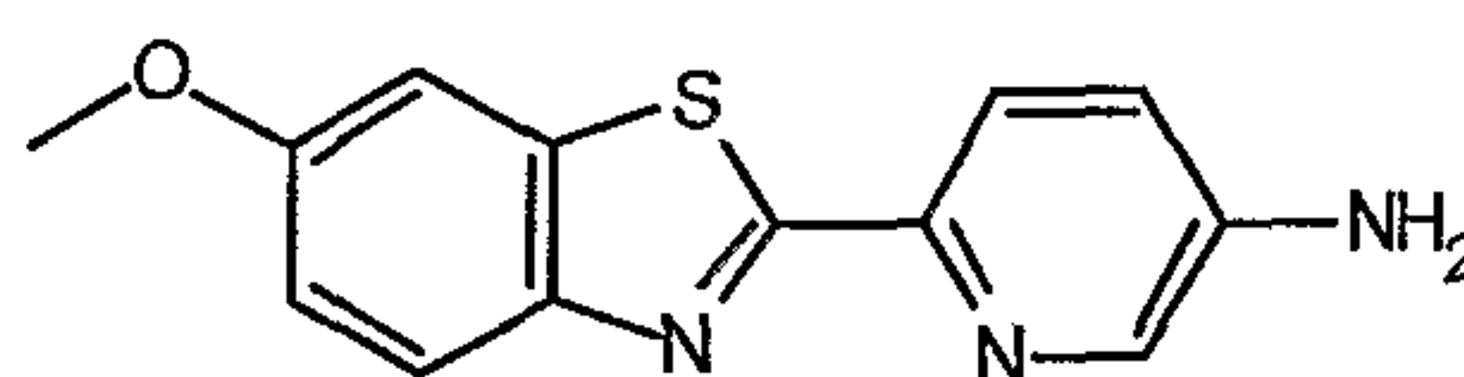
6-(6-methoxy-1,3-benzothiazol-2-yl)pyridin-3-amine
