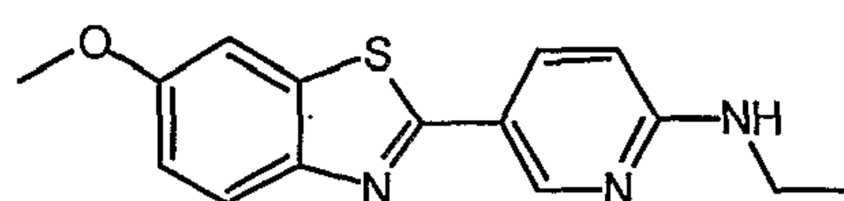
N-ethyl-5-(6-methoxy-1,3-benzothiazol-2-yl)pyridin-2-amine
