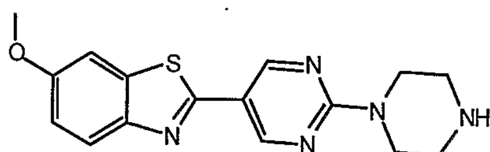
6-methoxy-2-(2-piperazin-1-yl)pyrimidin-5-yl)-1,3-benzothiazole
