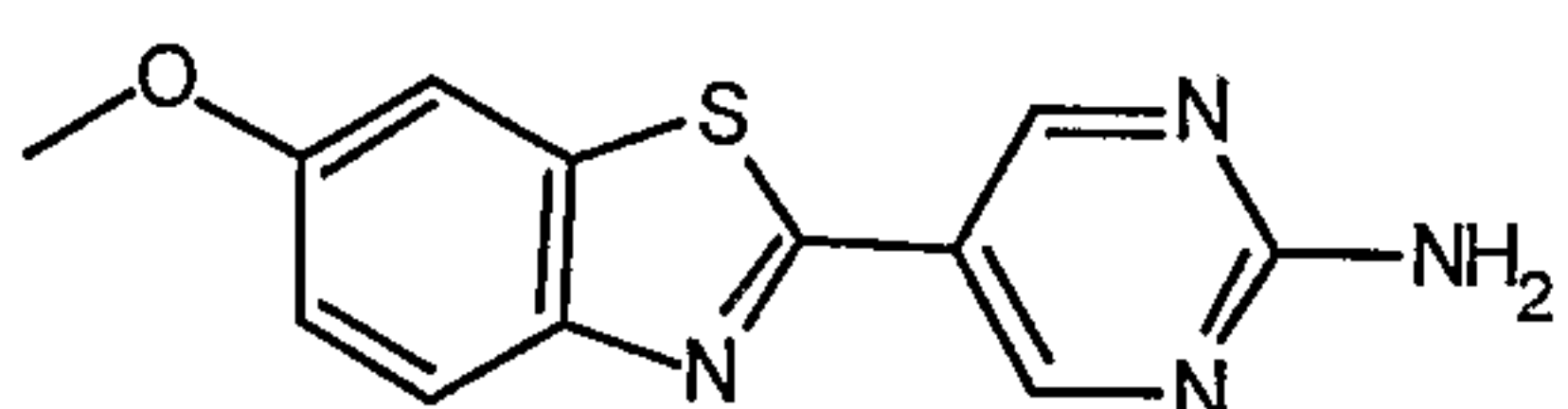
5-(6-methoxy-1,3-benzothiazol-2-yl)pyrimidin-2-amine
