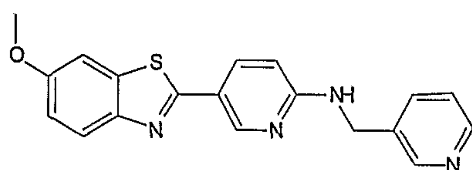
5-(6-Methoxy-1,3-benzothiazol-2-yl)-N-(pyridin-3-ylmethyl)pyridin-2-amine
