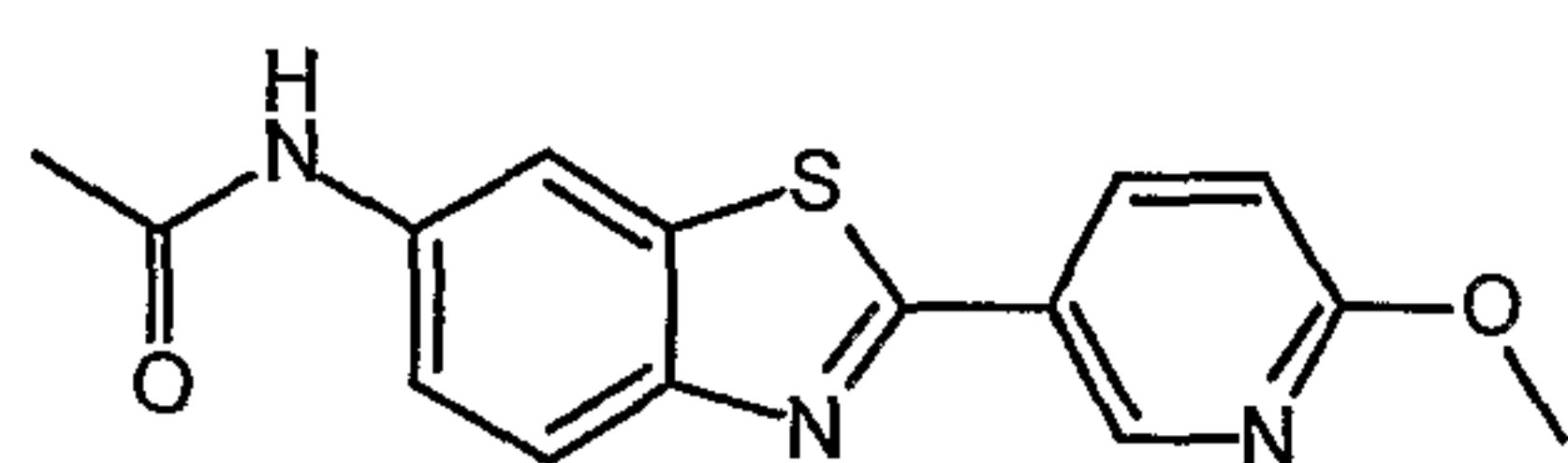
N-[2-(6-Methoxypyridin-3-yl)-1,3-benzothiazol-6-yl]acetamide
