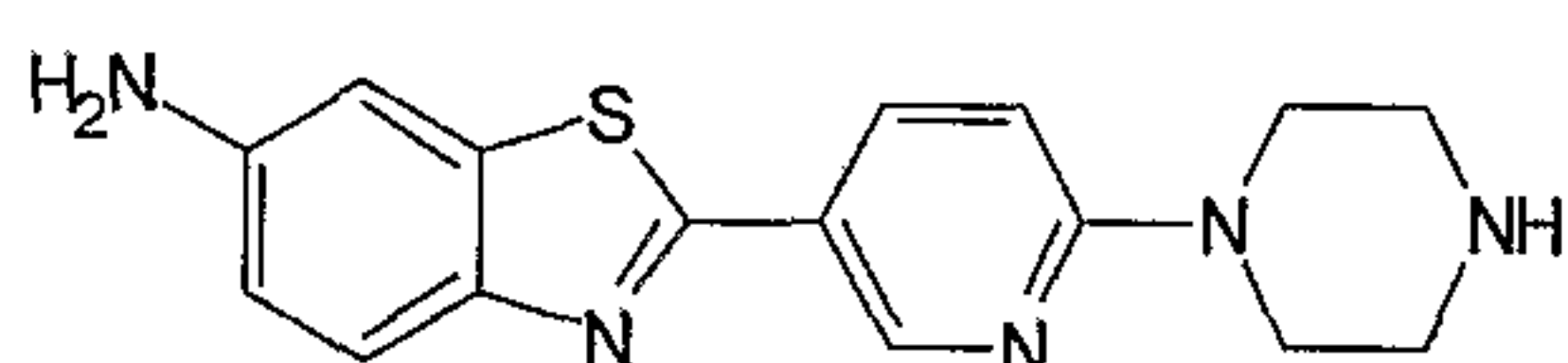
2-(6-Piperazin-1-ylpyridin-3-yl)-1,3-benzothiazol-6-amine
