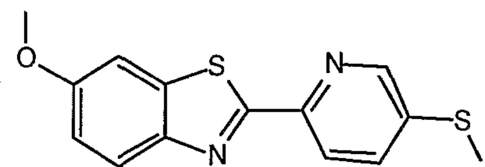
6-methoxy-2-[5-(methylthio)pyridin-2-yl]-1,3-benzothiazole
