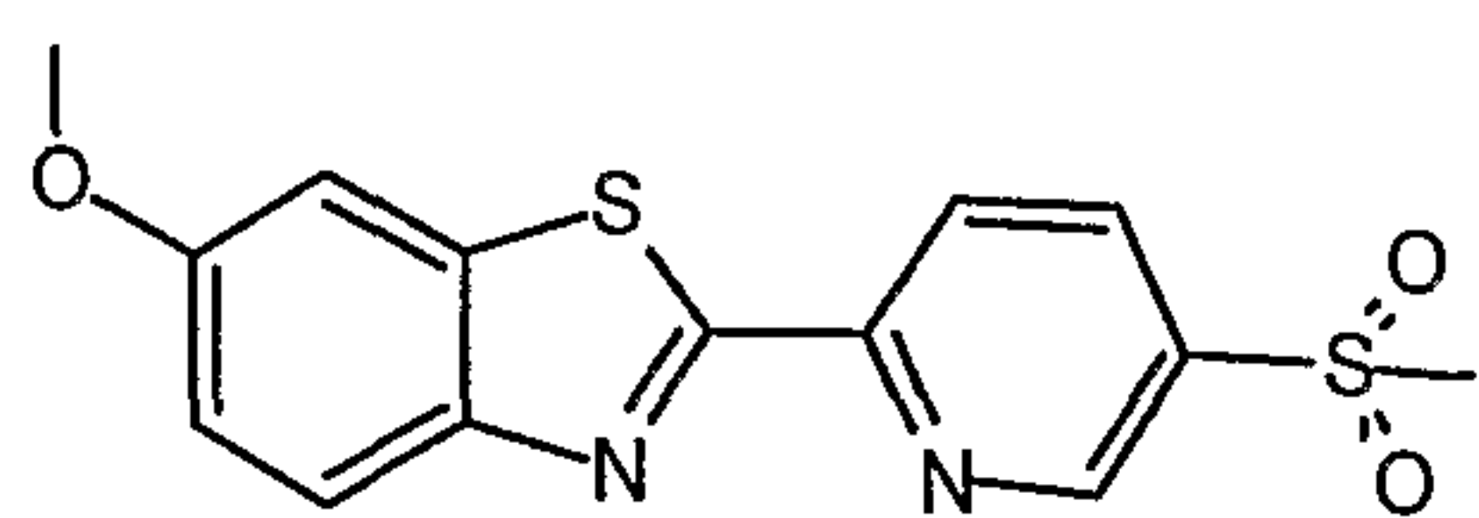
6-methoxy-2-[5-(methylsulfonyl)pyridin-2-yl]-1,3-benzothiazole
