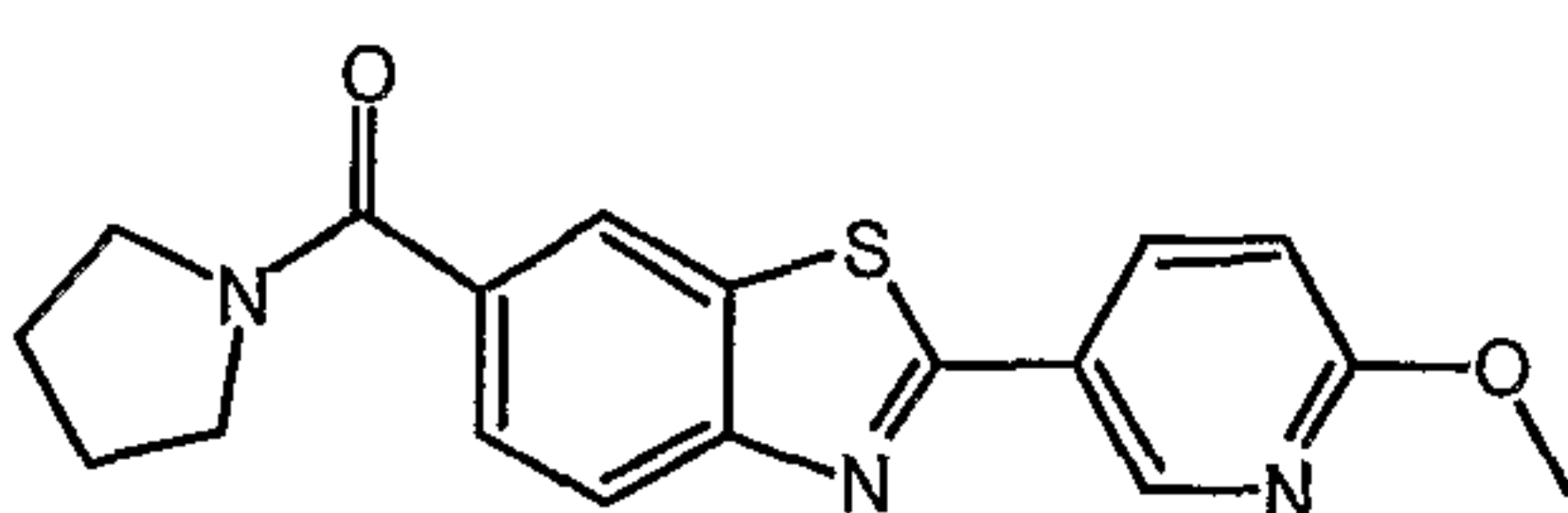
2-(6-Methoxypyridin-3-yl)-6-(pyrrolidin-1-ylcarbonyl)-1,3-benzothiazole
