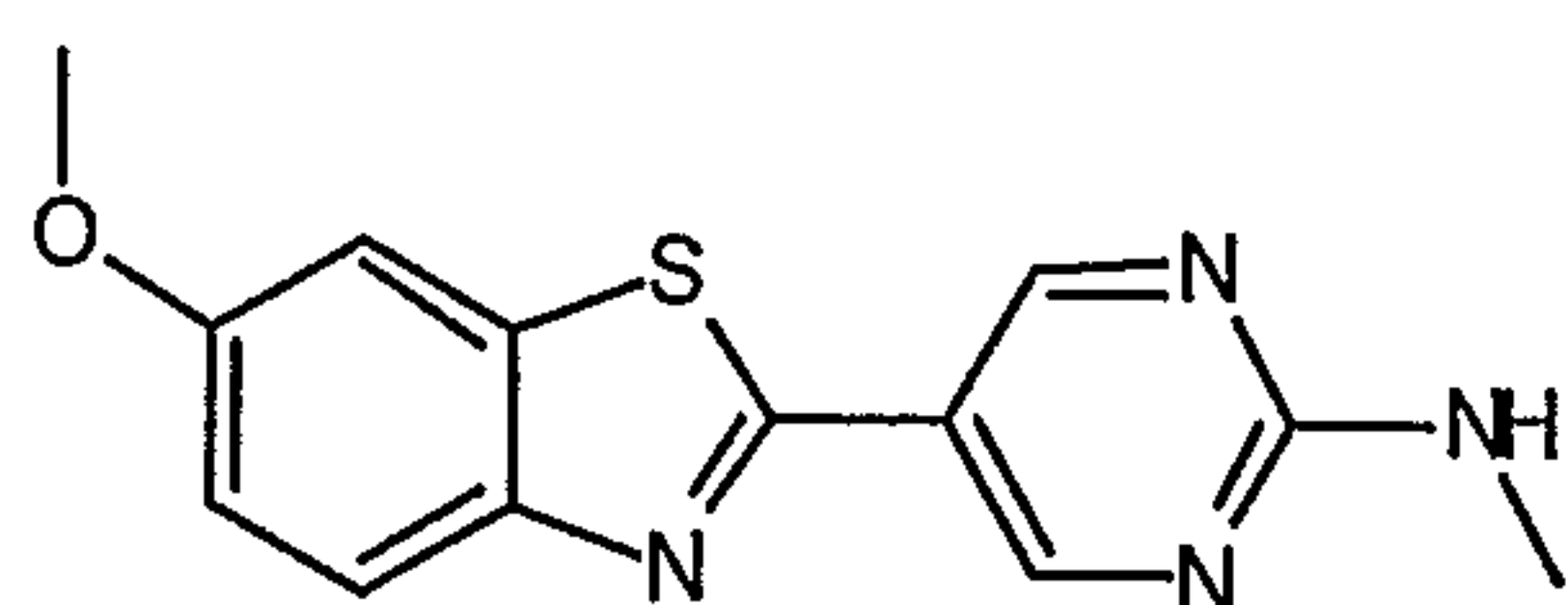
5-(6-methoxy-1,3-benzothiazol-2-yl)-N-methylpyrimidin-2-amine
