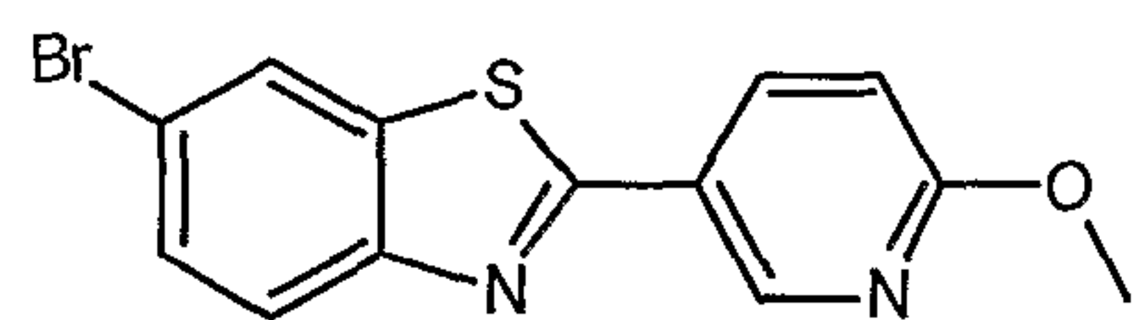
6-Bromo-2-(6-methoxypyridin-3-yl)-1,3-benzothiazole
