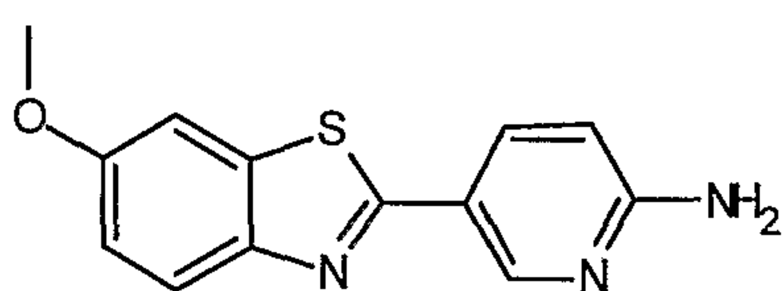
5-(6-Methoxy-1,3-benzothiazol-2-yl)pyridin-2-amine
