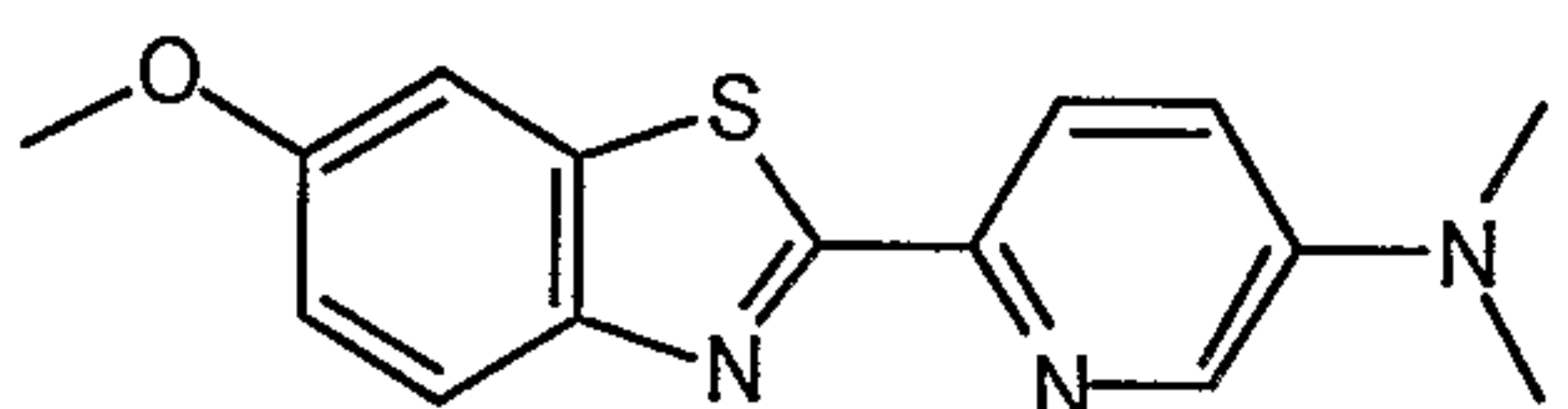
6-(6-methoxy-1,3-benzothiazol-2-yl)-N,N-dimethylpyridin-3-amine
