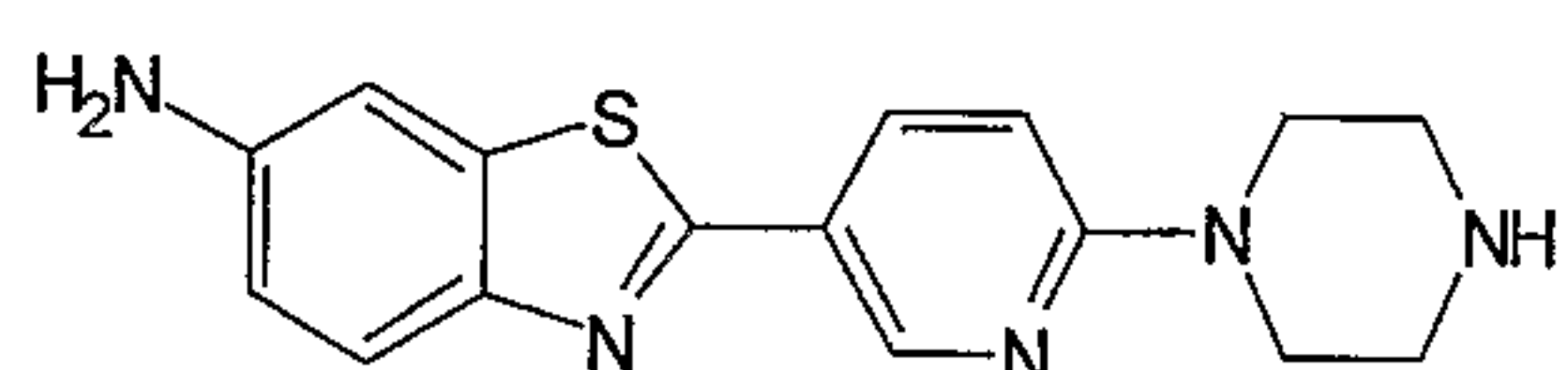
2-(6-Piperazin-1-ylpyridin-3-yl)-1,3-benzothiazol-6-amine
