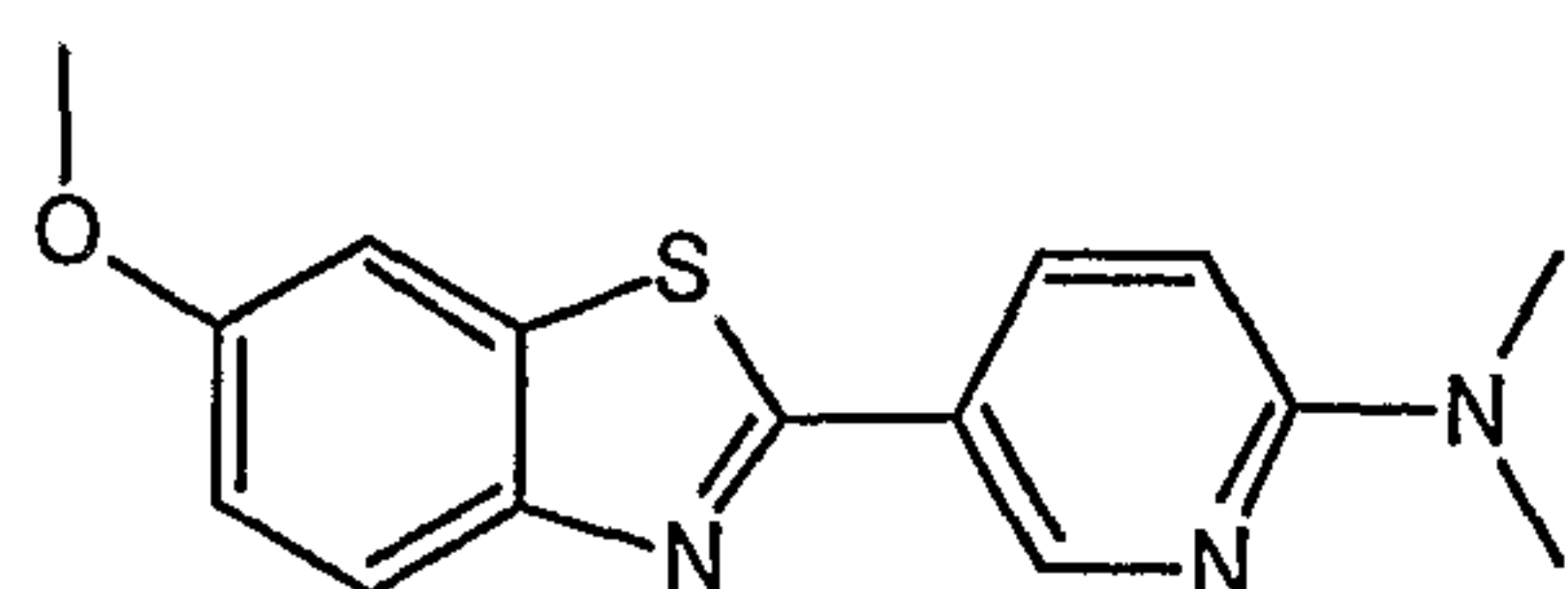
5-(6-methoxy-1,3-benzothiazol-2-yl)-N,N-dimethylpyridin-2-amine
