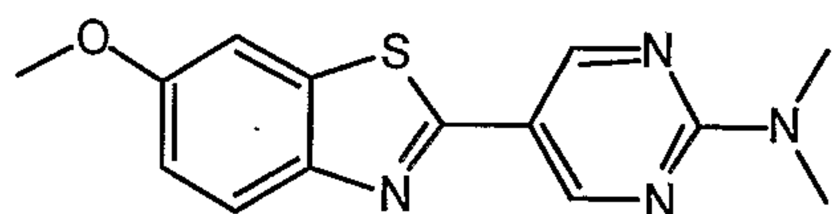
5-(6-methoxy-1,3-benzothiazol-2-yl)-N,N-dimethylpyrimidin-2-amine
