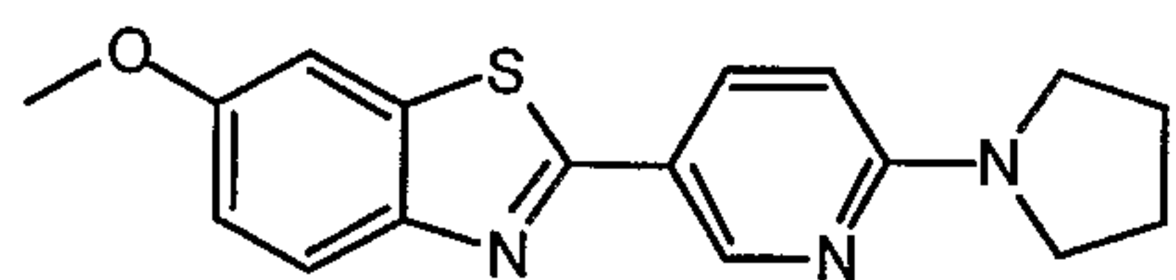
6-methoxy-2-(6-pyrrolidin-1-ylpyridin-3-yl)-1,3-benzothiazole
