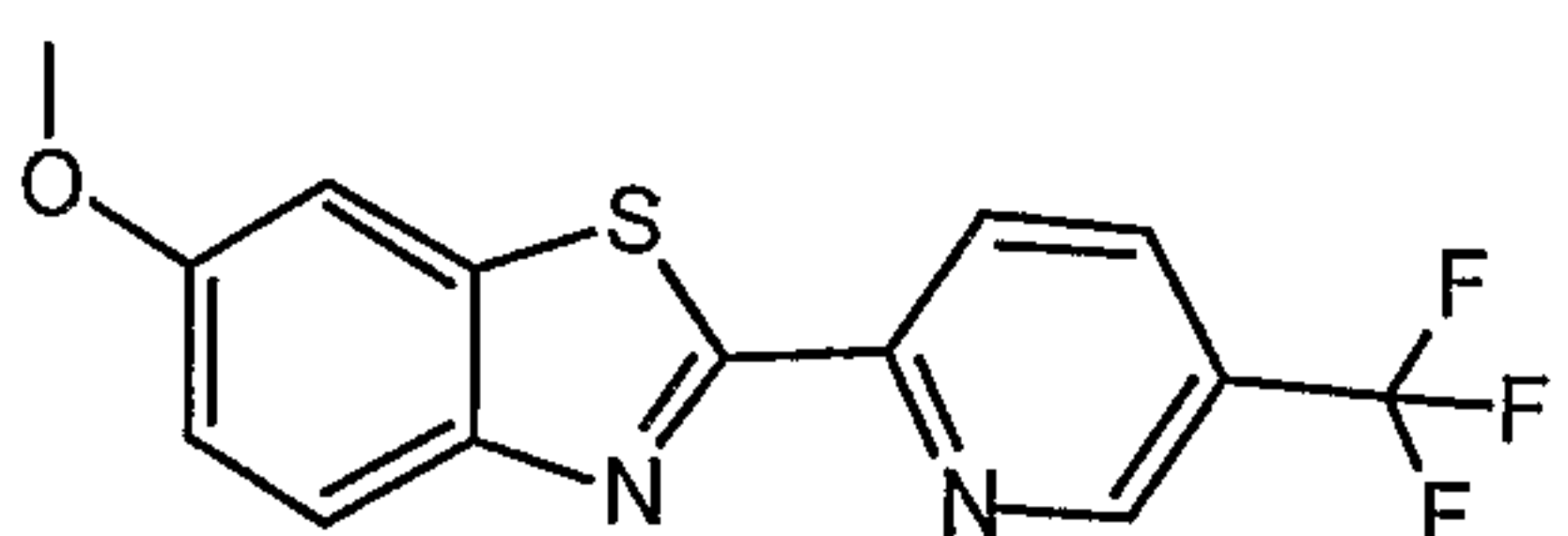
6-methoxy-2-[5-(trifluoromethyl)pyridin-2-yl]-1,3-benzothiazole
