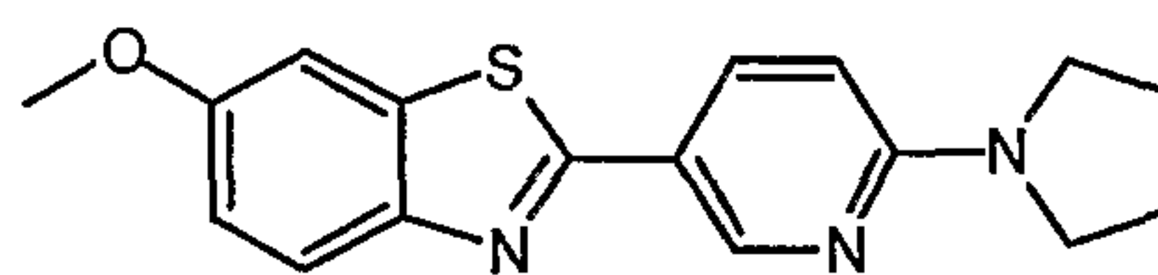
6-methoxy-2-(6-pyrrolidin-1-ylpyridin-3-yl)-1,3-benzothiazole
