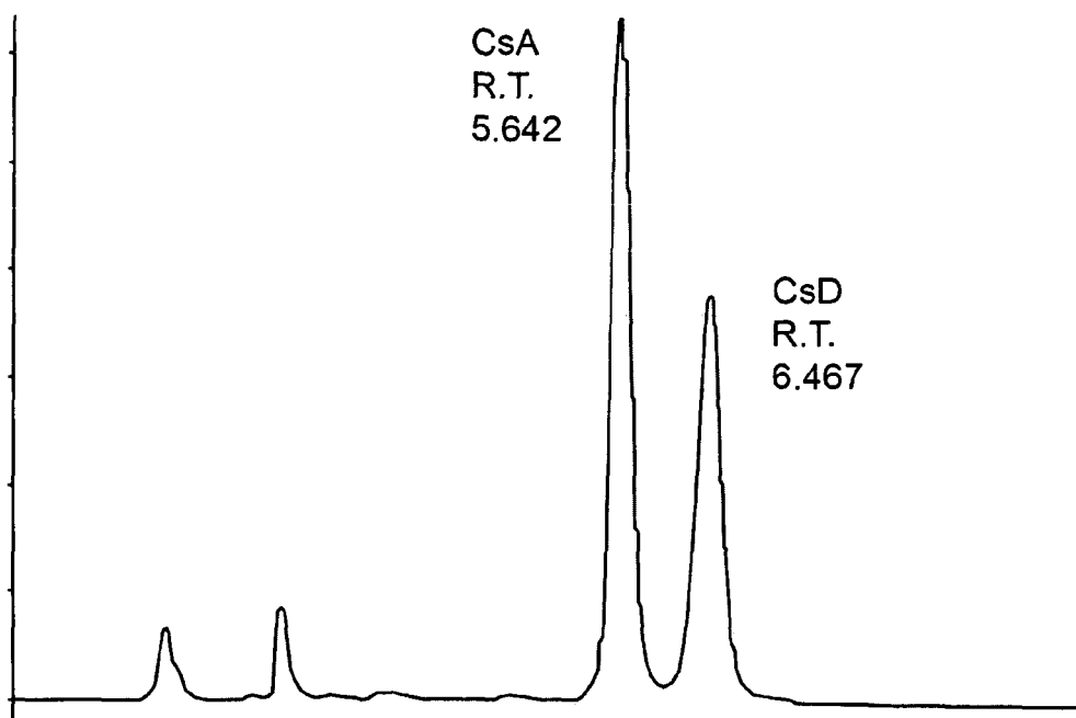
Fig. 9 CsA and CsD HPLC chromatogram
