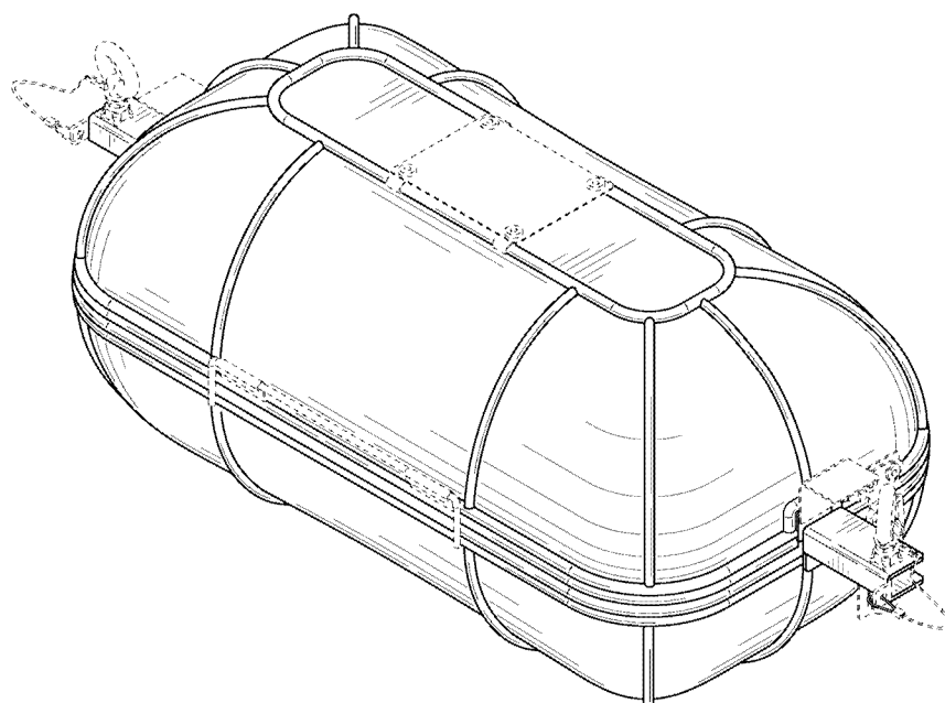
【立體圖】
