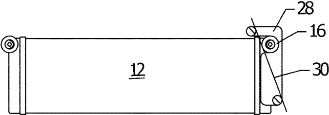
FIG. 6 SECTION A-A
