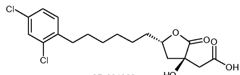
SB-204990
