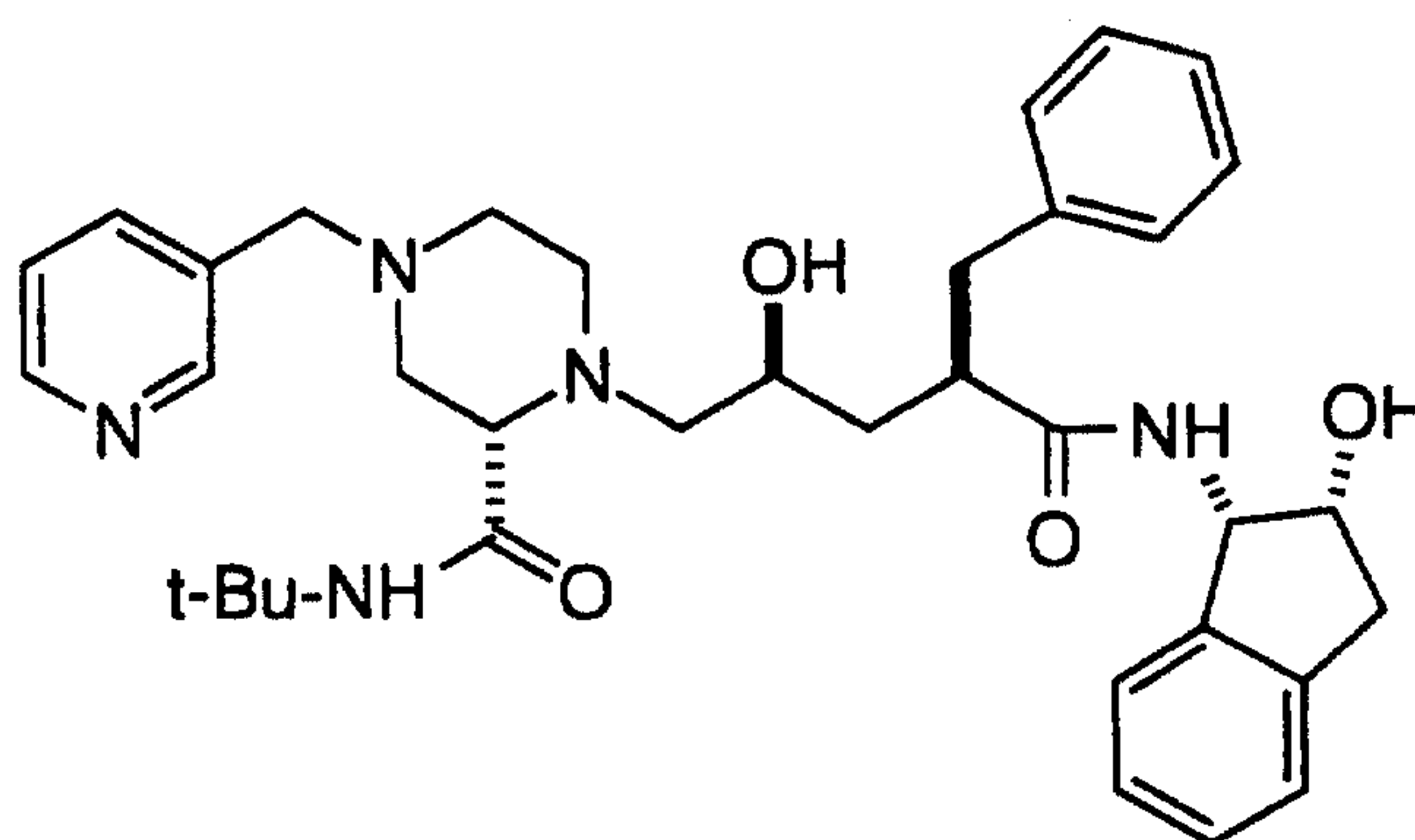
Indinavir
