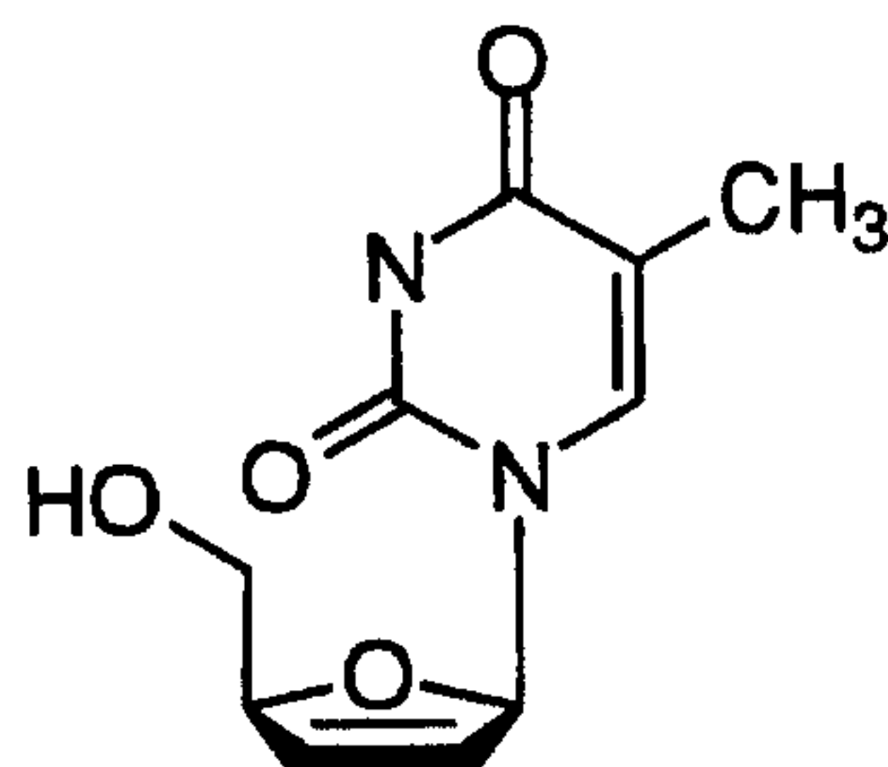
Stavudine
