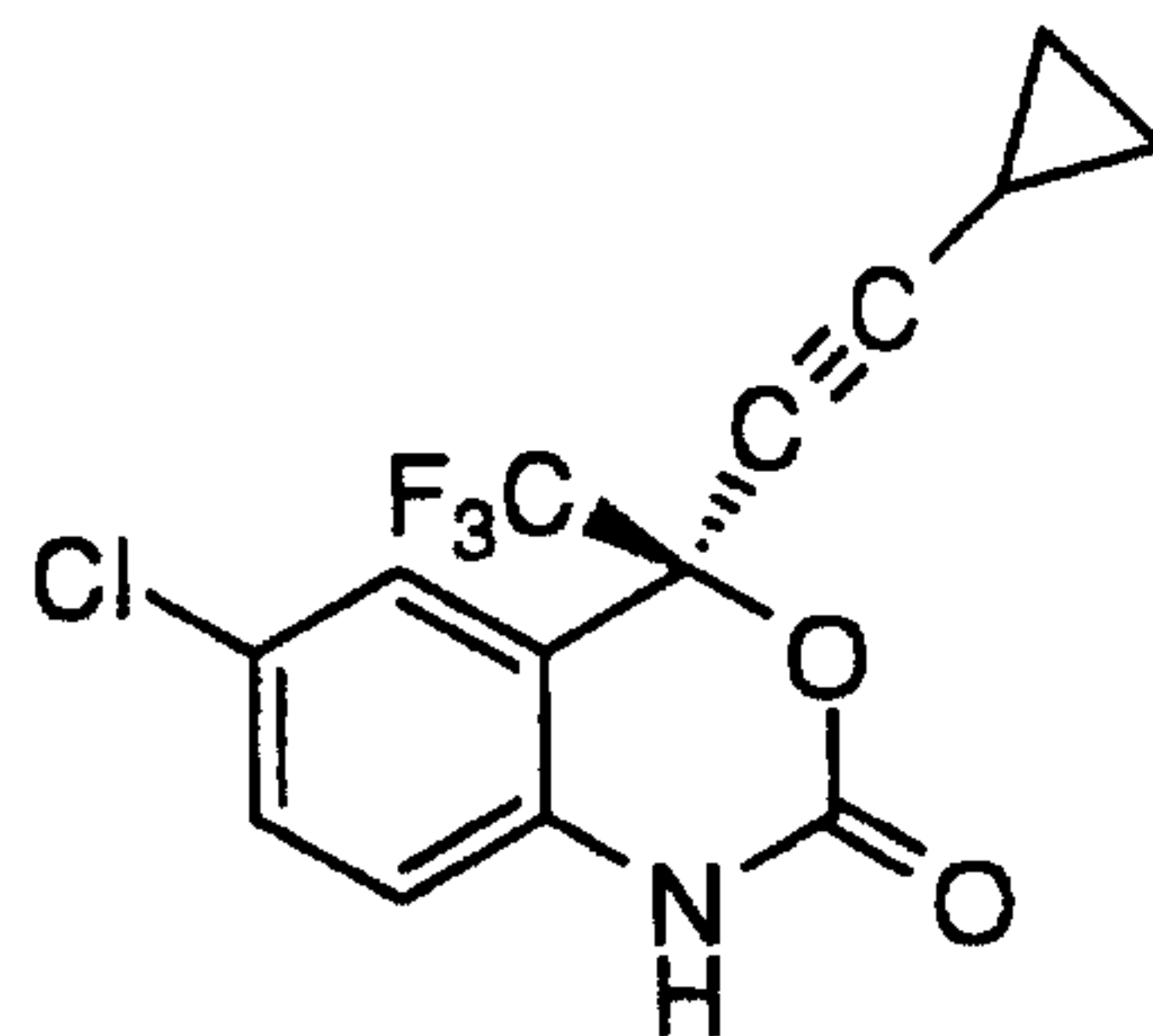
DMP-266
