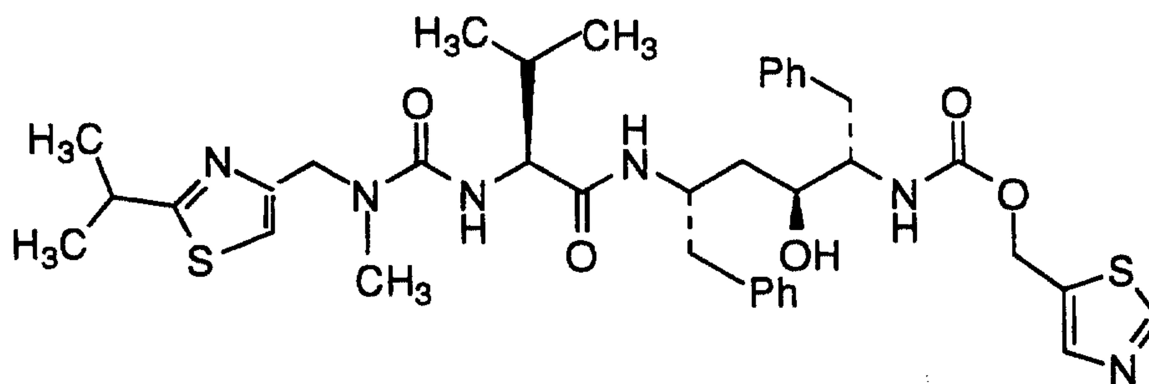
Ritonavir
