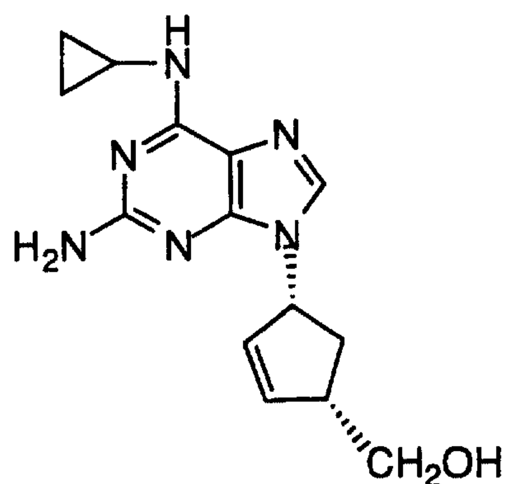
Abacavir
