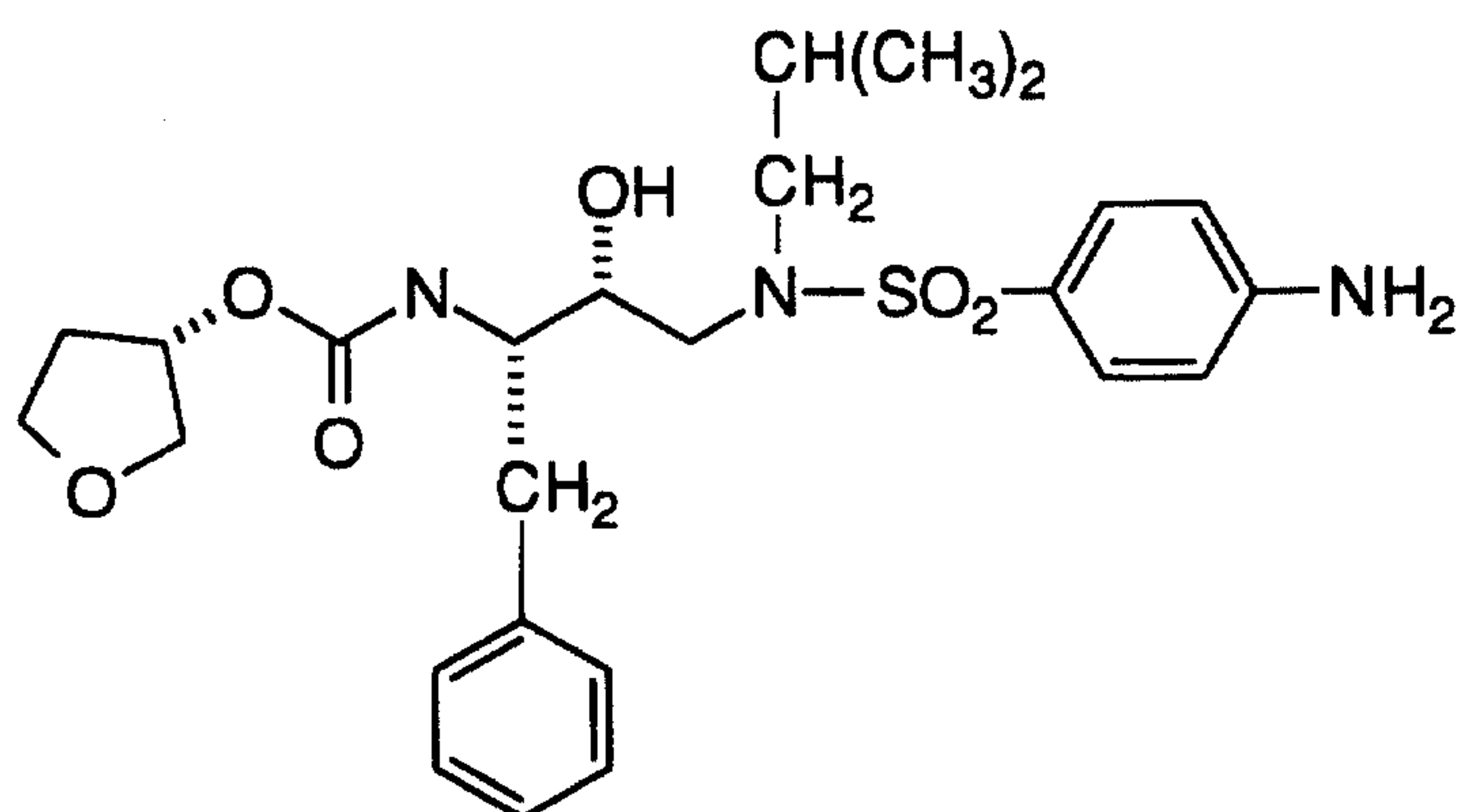
141-W94
