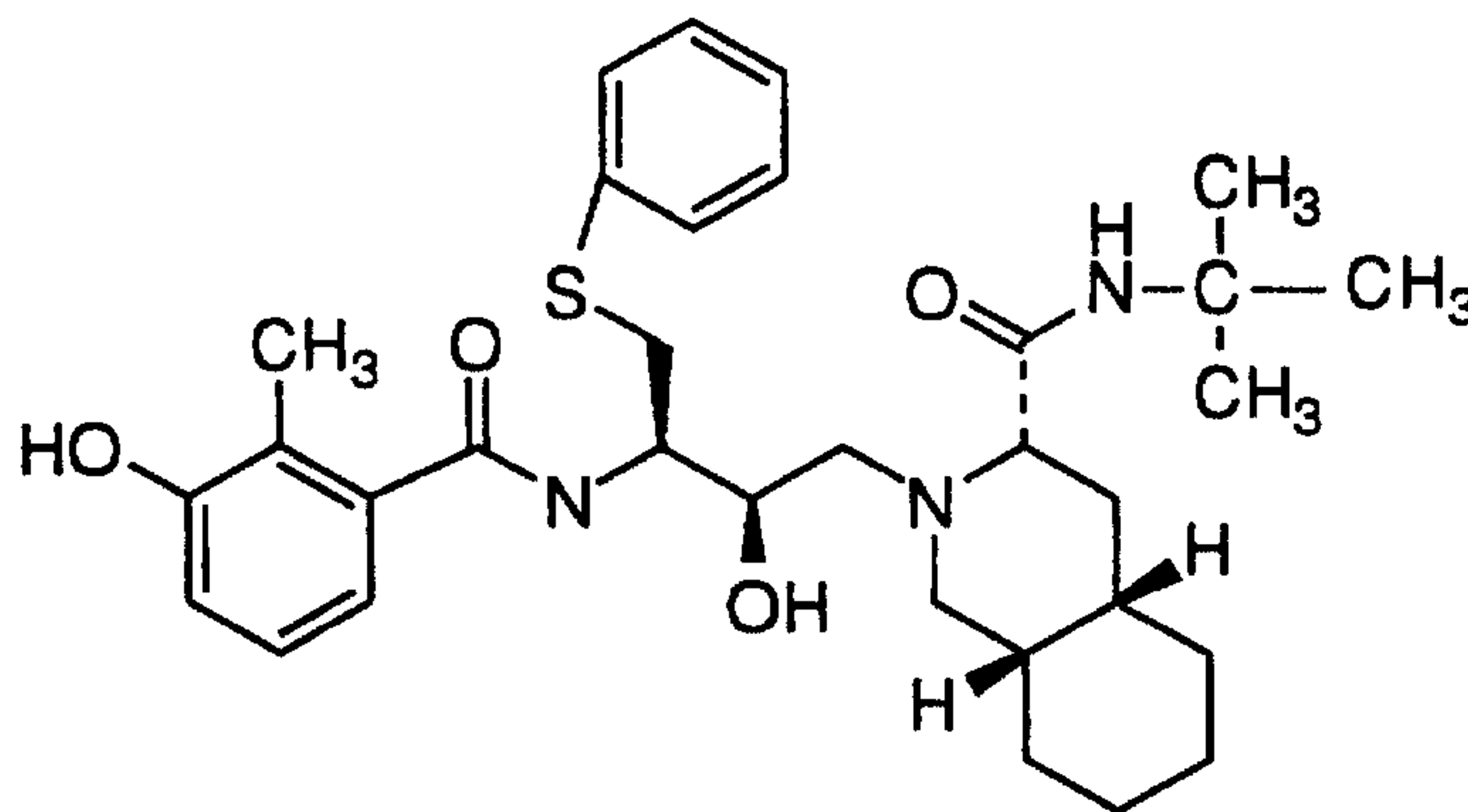
Nelfinavir
