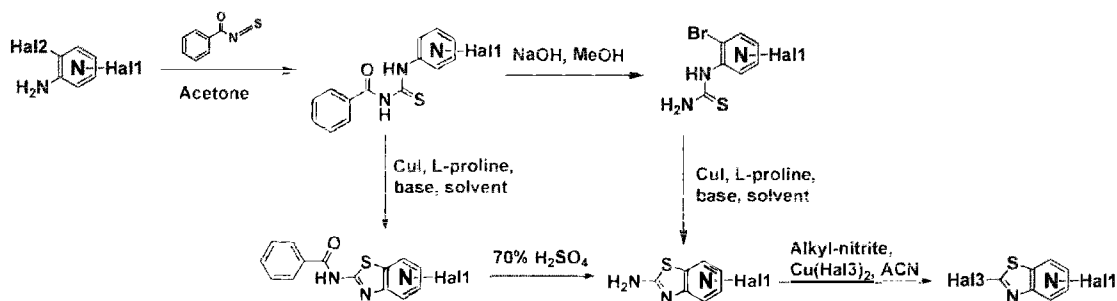
Scheme 1a
