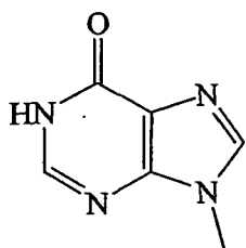
Inosine
