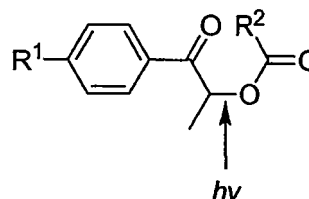
p-alkoxy
