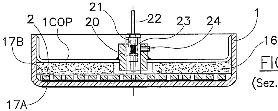
FIG. 6 (Sez. A-A)
