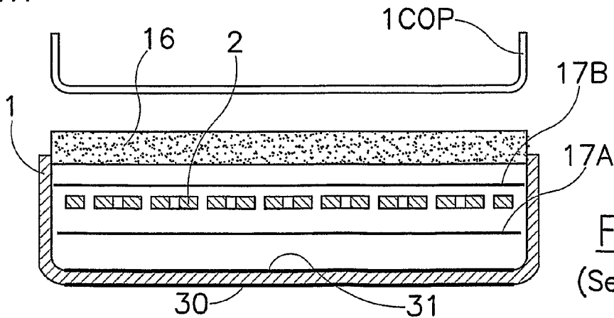
FIG. 7 (Sez. B-B)
