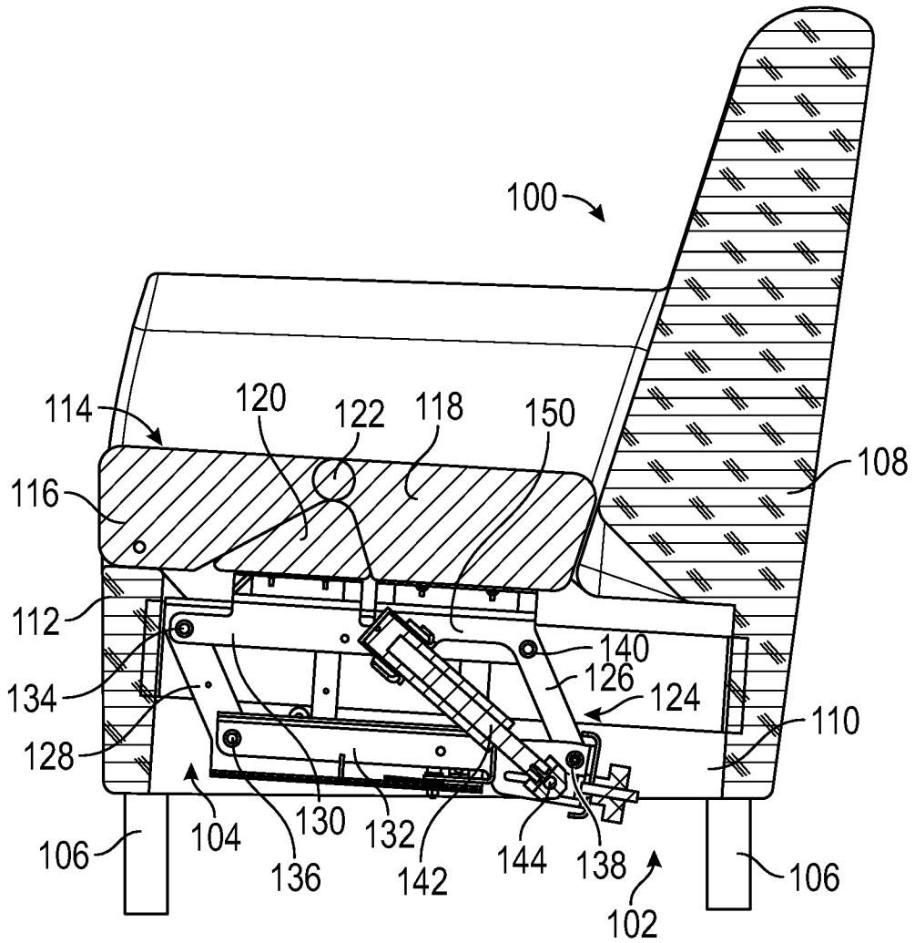
SECTION 3-3 SCALE 1 : 6 FIG. 3
