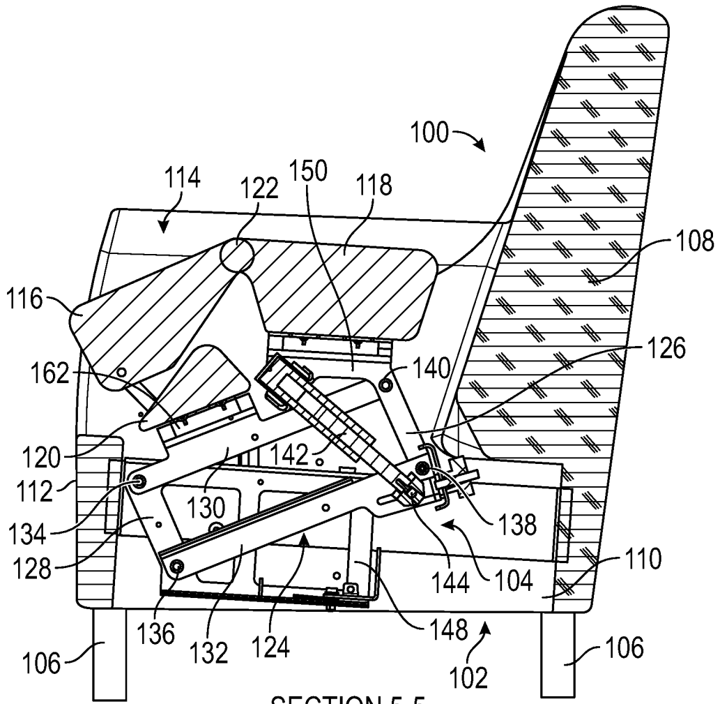
SECTION 5-5 SCALE 1 : 6 FIG. 5
