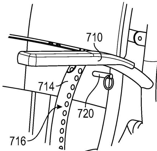
DETAIL I SCALE 1:4 FIG. 54B
