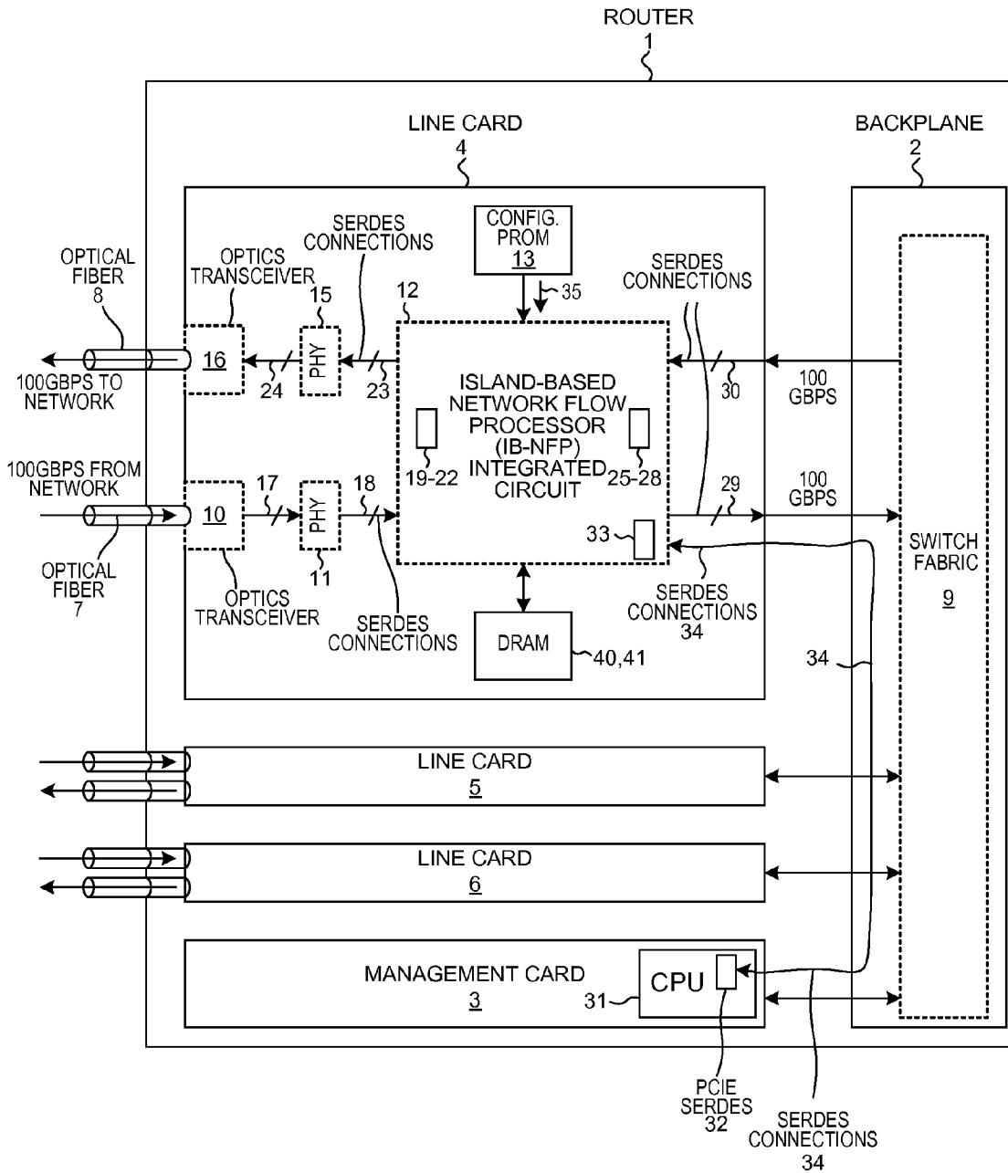
MPLS ROUTER FIG. 1
