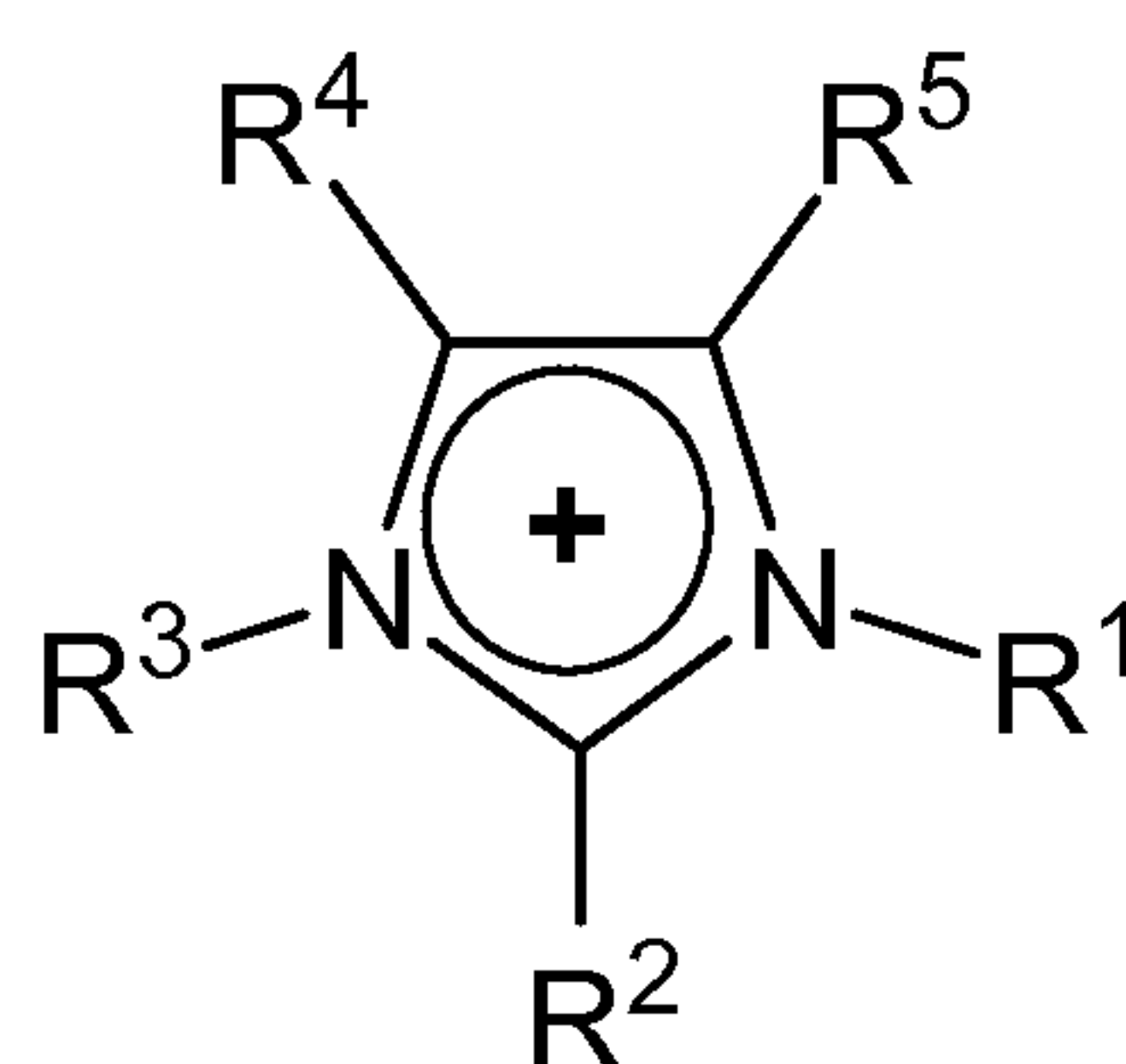
Imidazolium;
