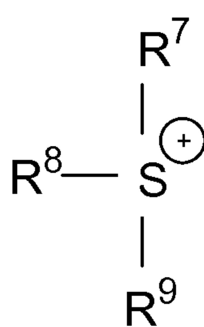
15 Sulfonium;
