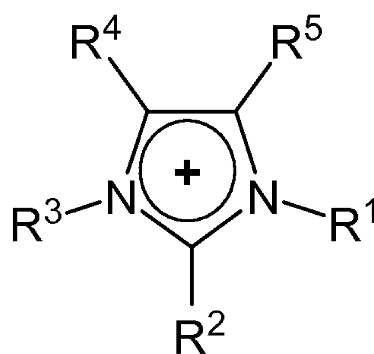
Imidazolium
