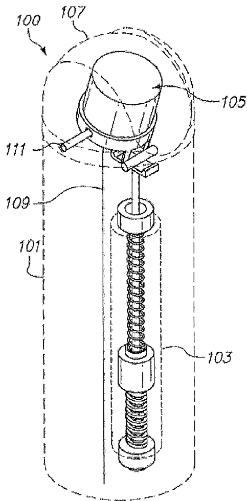
PRIOR ART Fig. 1A
