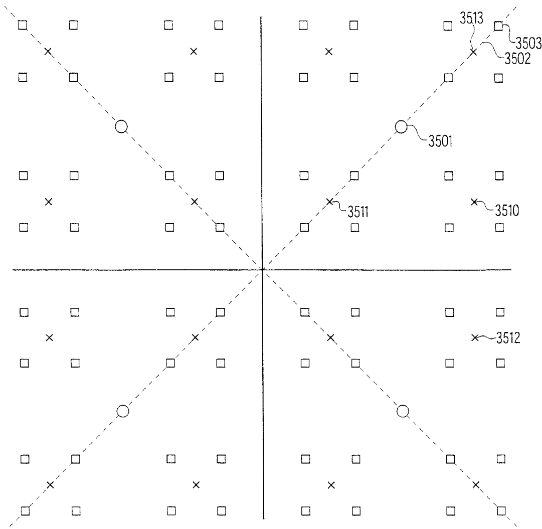
QAM-64
