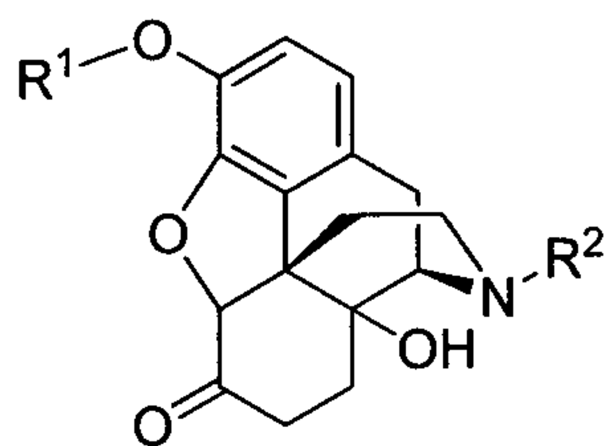
(IV)
