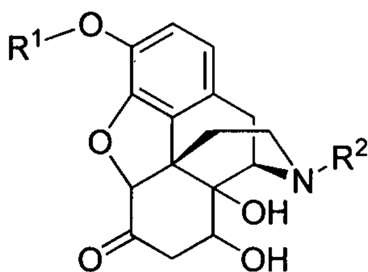
(III)
