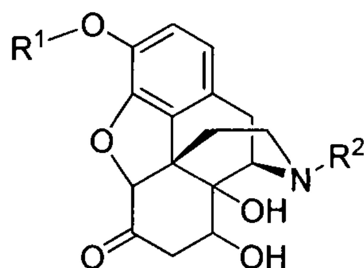
(III)
