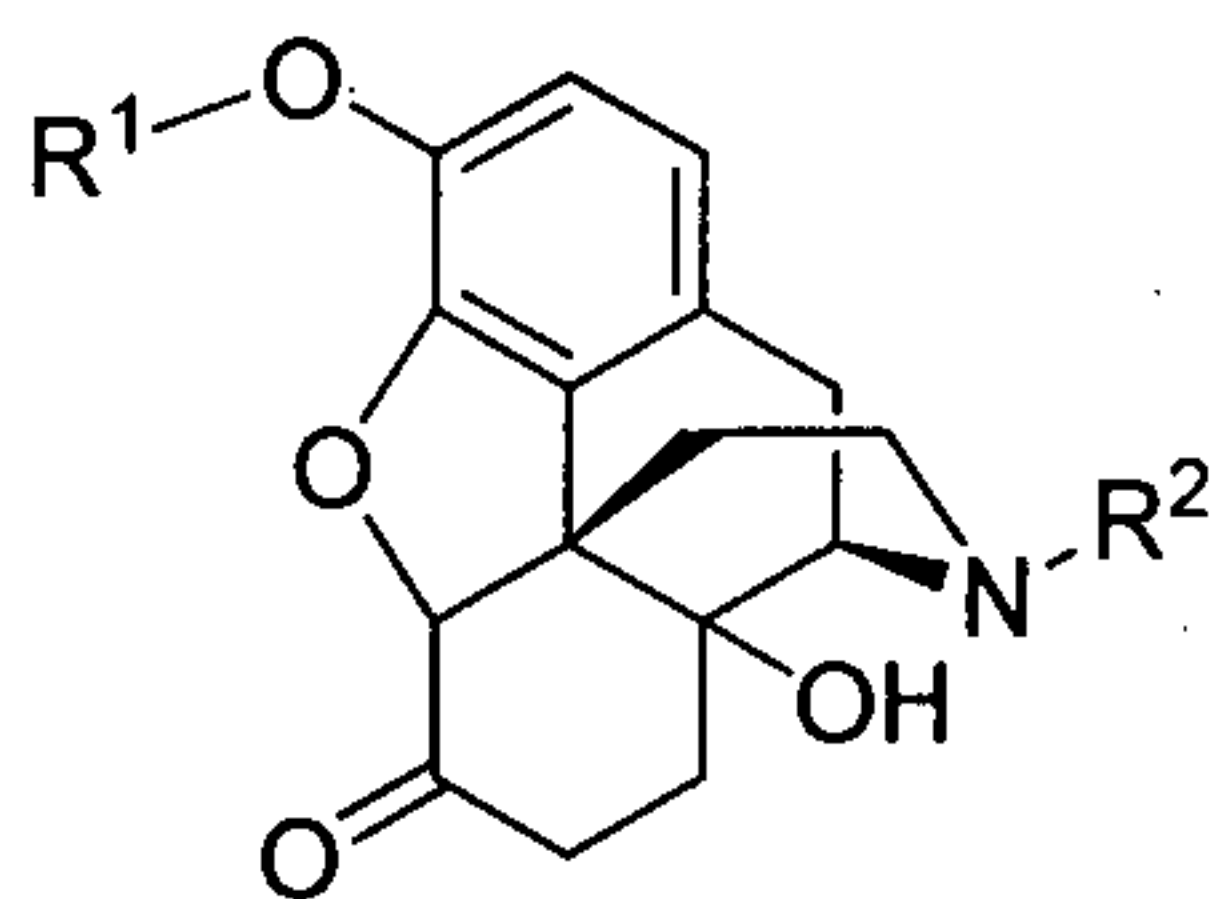
(IV)
