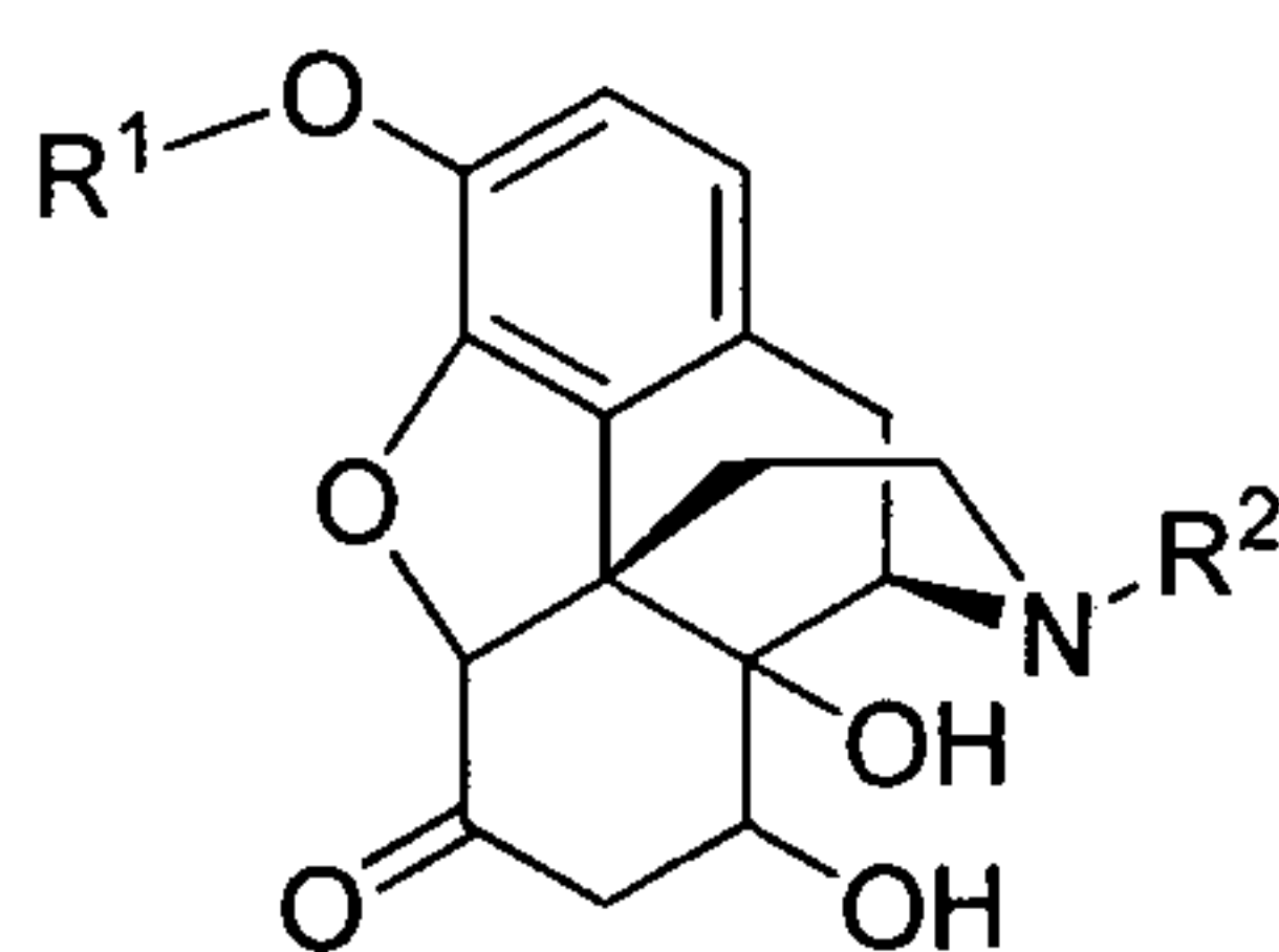
(III)
