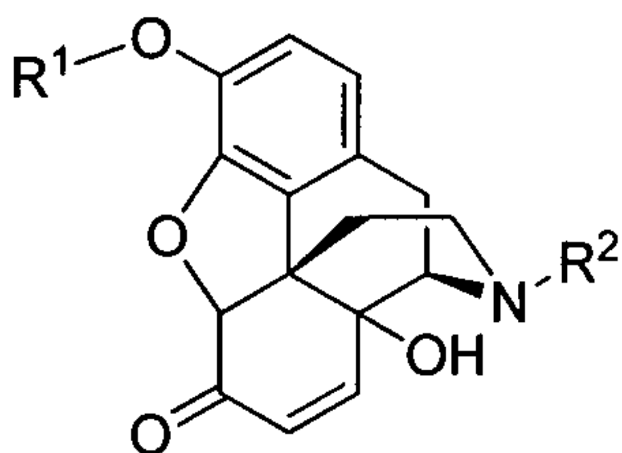
(II)
