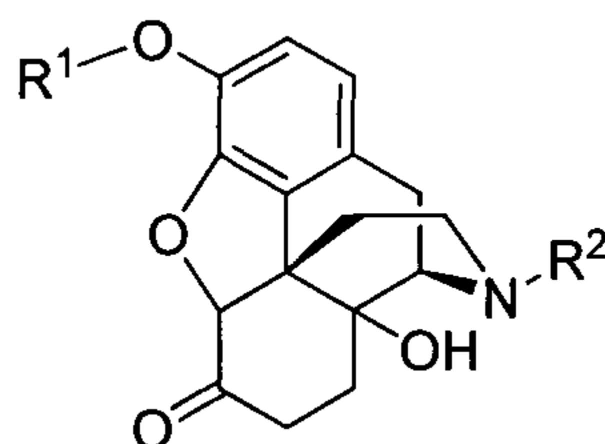
(IV)
