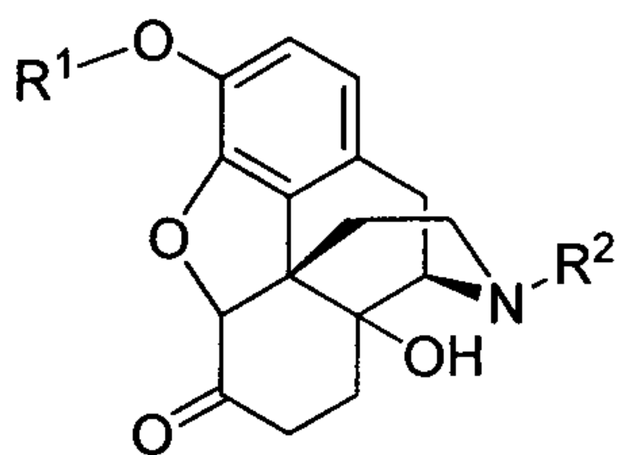
(IV)
