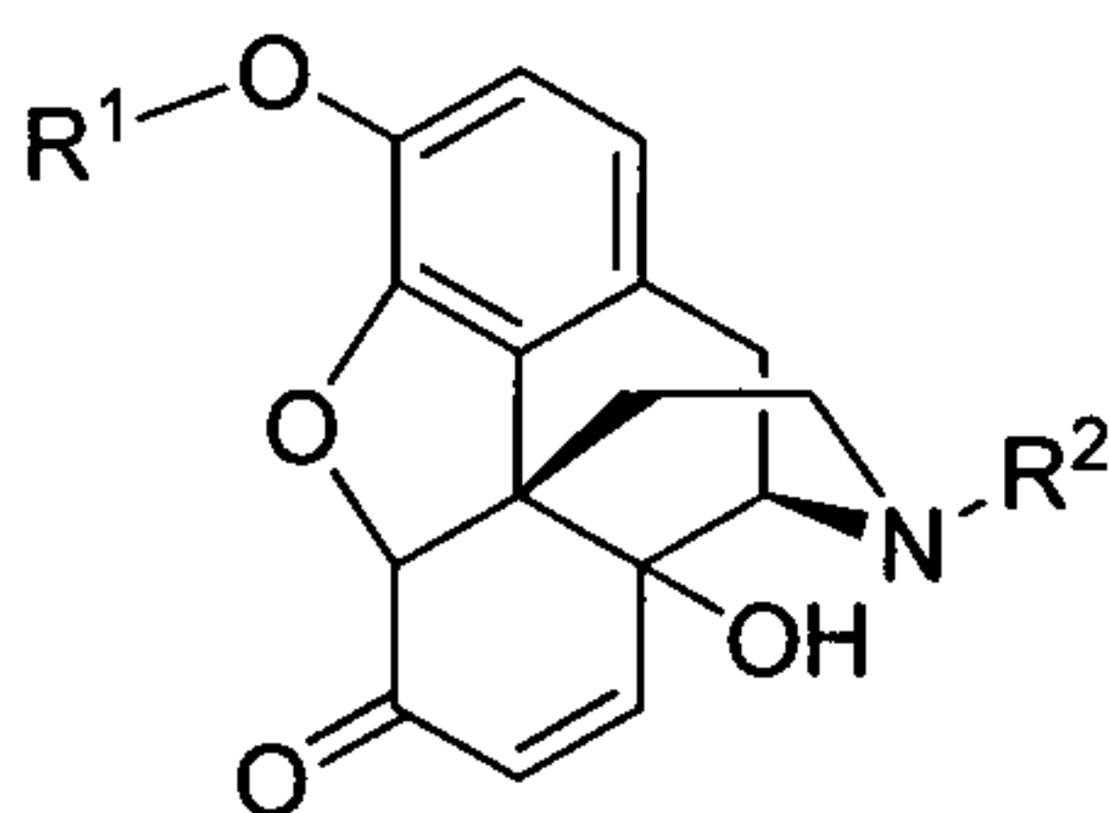
(II)
