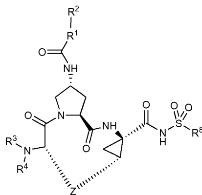
(VIIIe)
