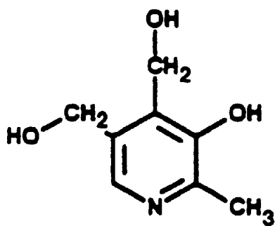
Pyridoxine
