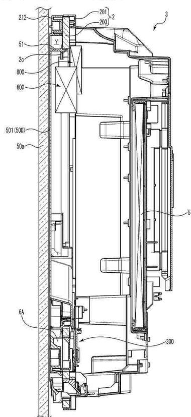
【图 10-4】 A-A 断面图
