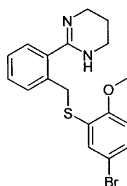
Compound IZ
