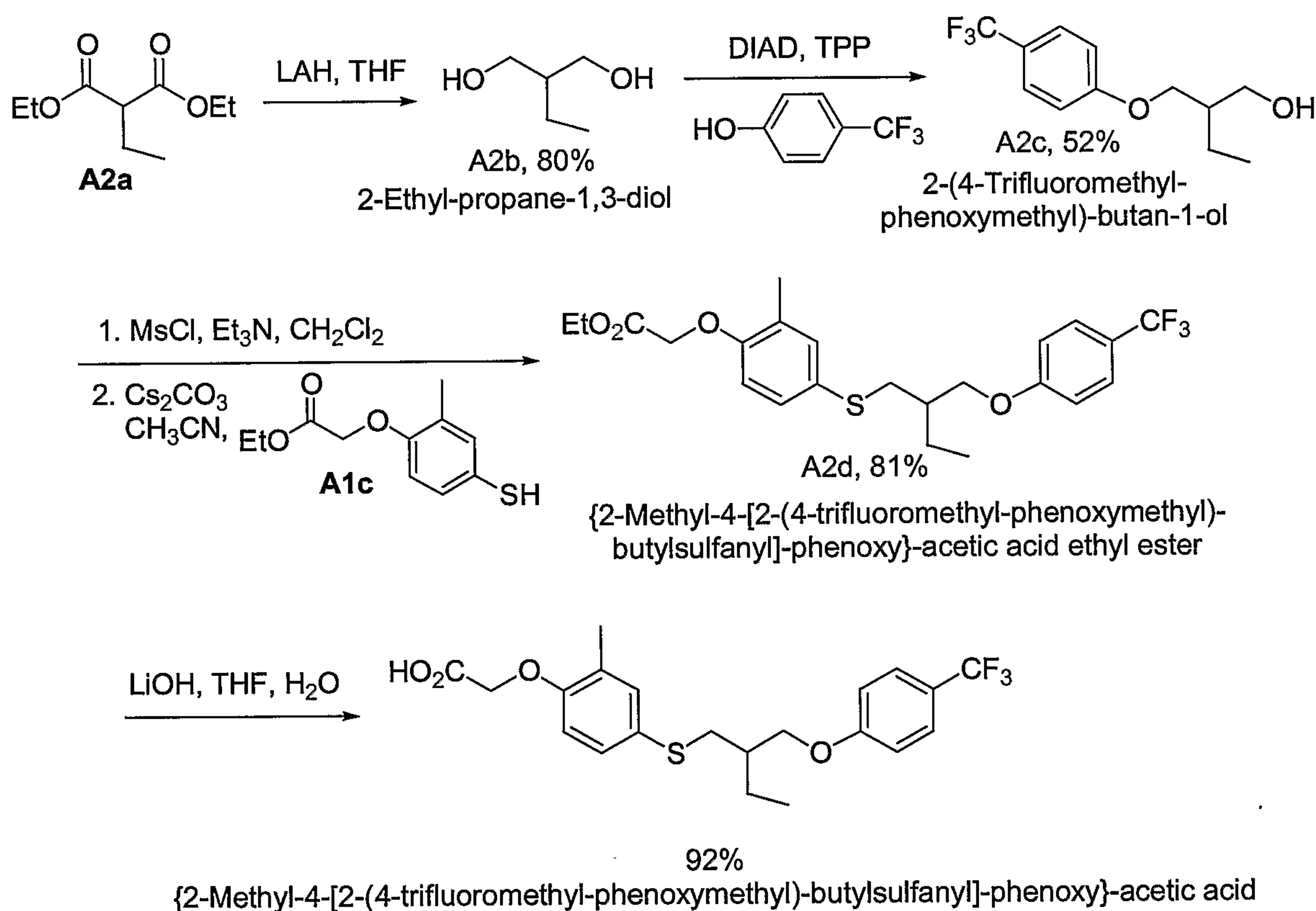
Scheme A2
