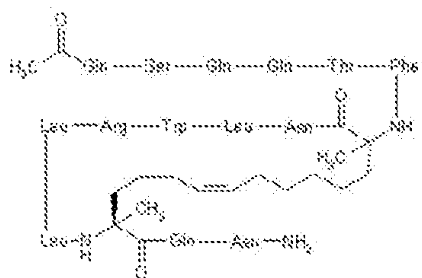
SAH-p53-8
