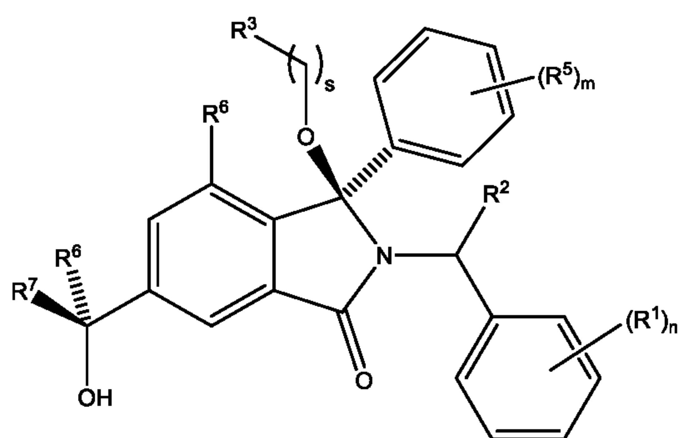
Diastereoisomer 2A
