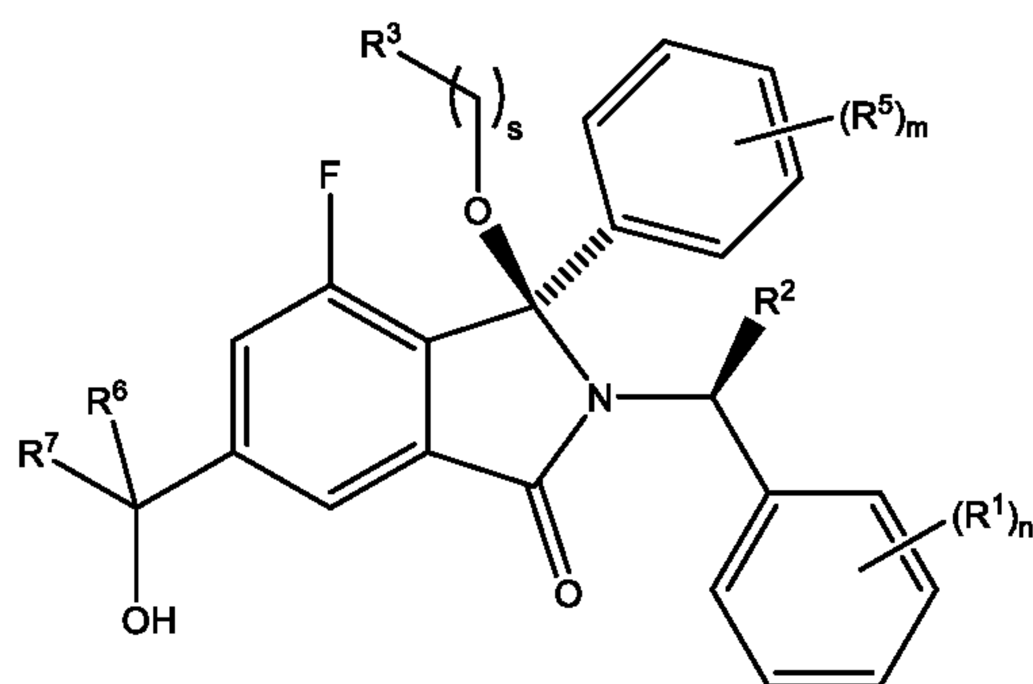
Diastereoisomer 1A
