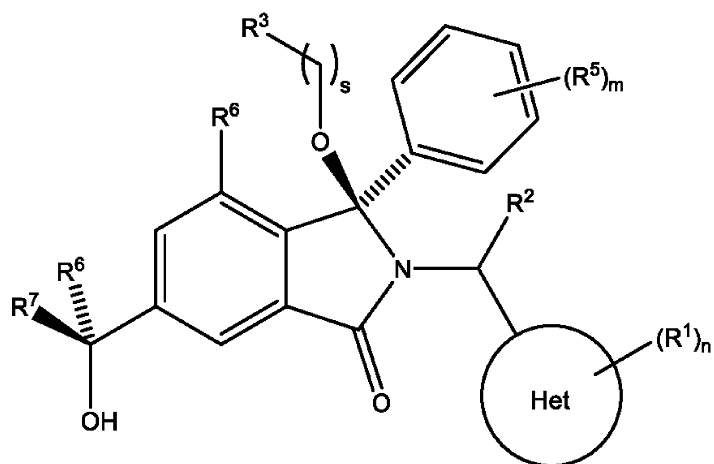
Diastereoisomer 2A
