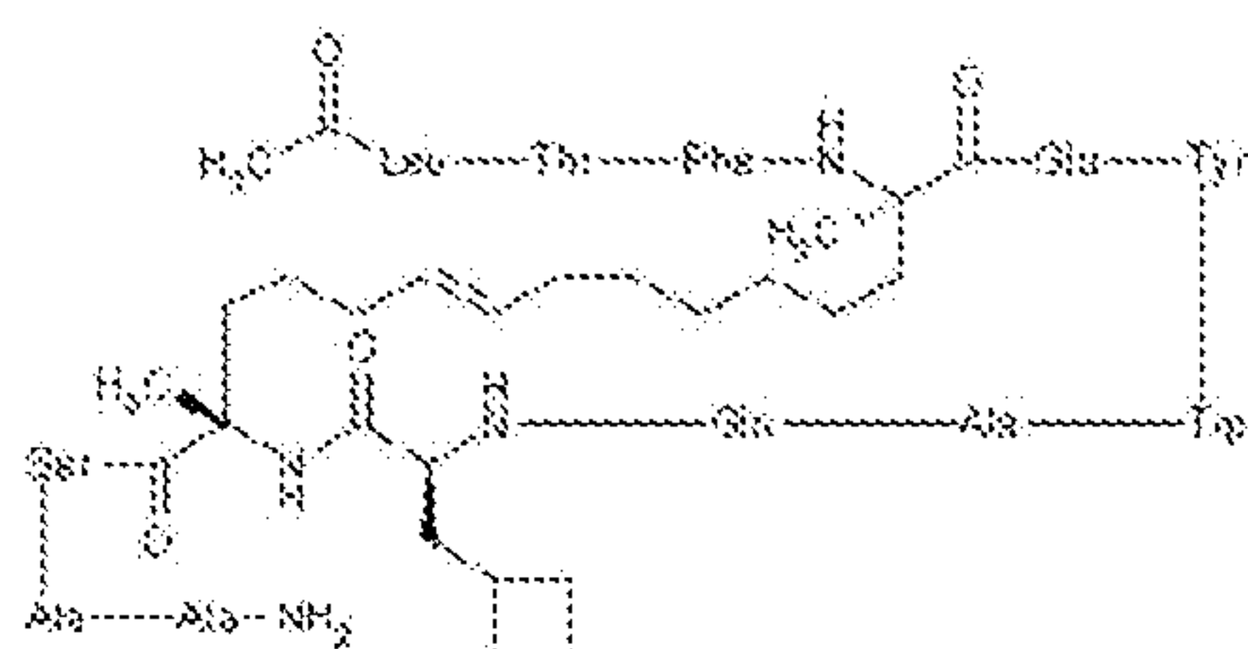
ATSP-7041
