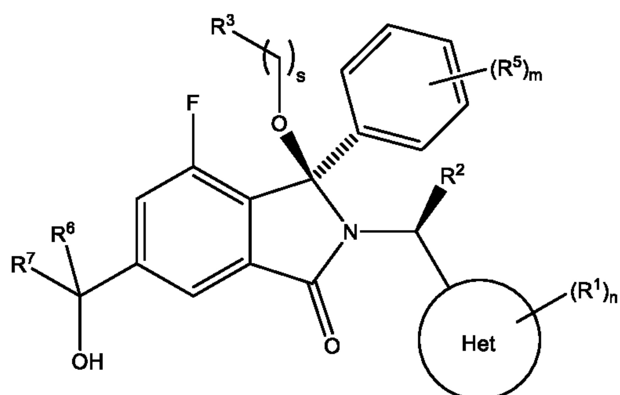
Diastereoisomer 1A
