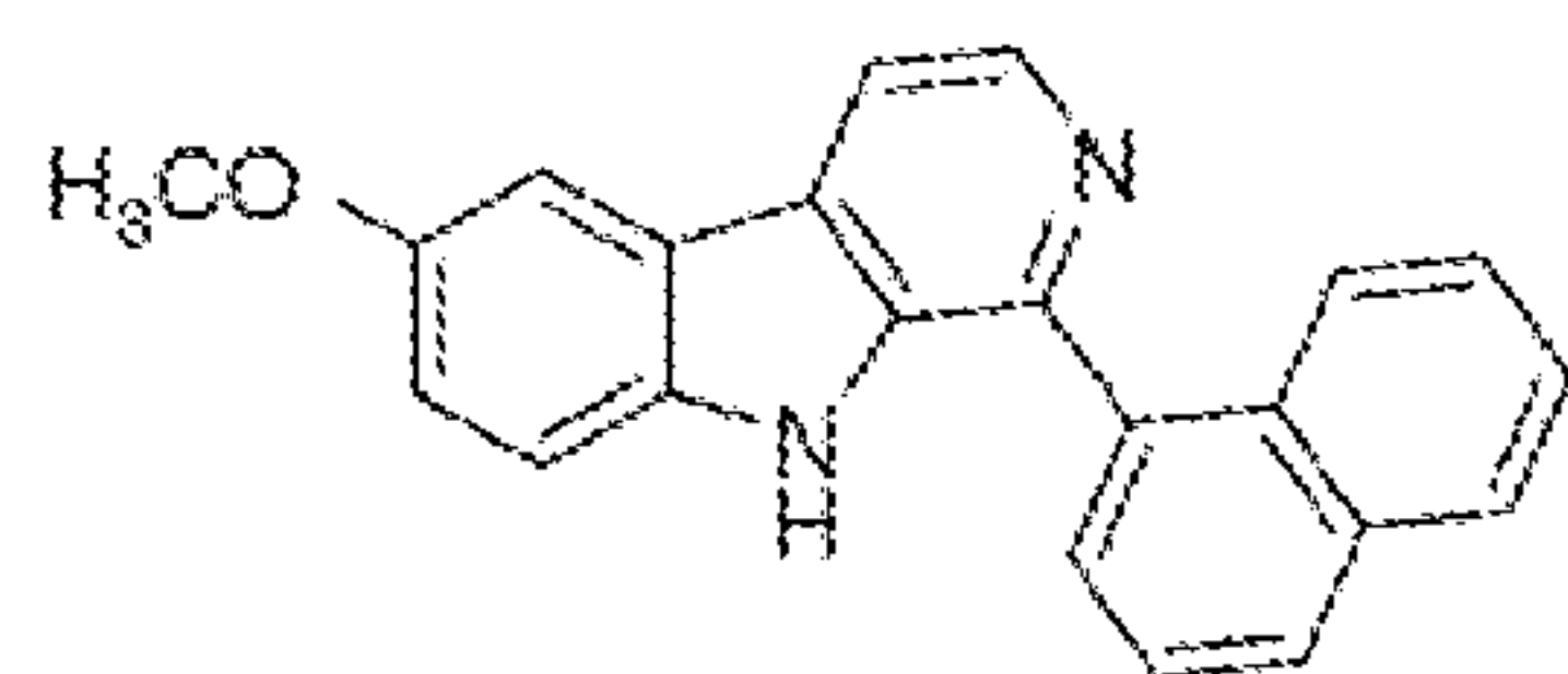
SP-141
