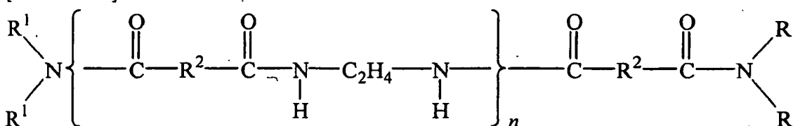
[Chem. 3]
