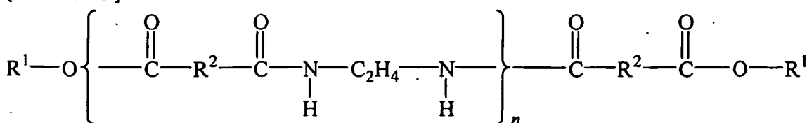
[Chem. 5]
