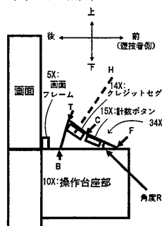
(2) メダル数表示ユニット 断面の概念図
