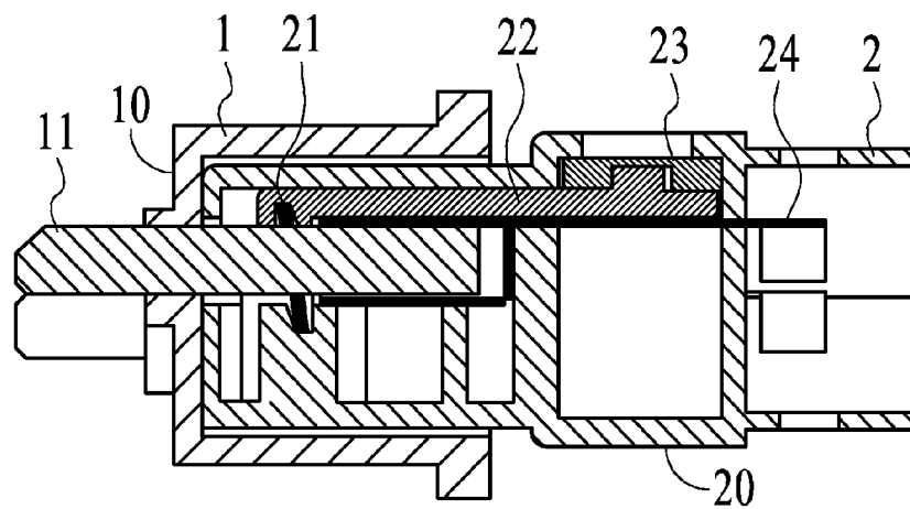
Section D-D
