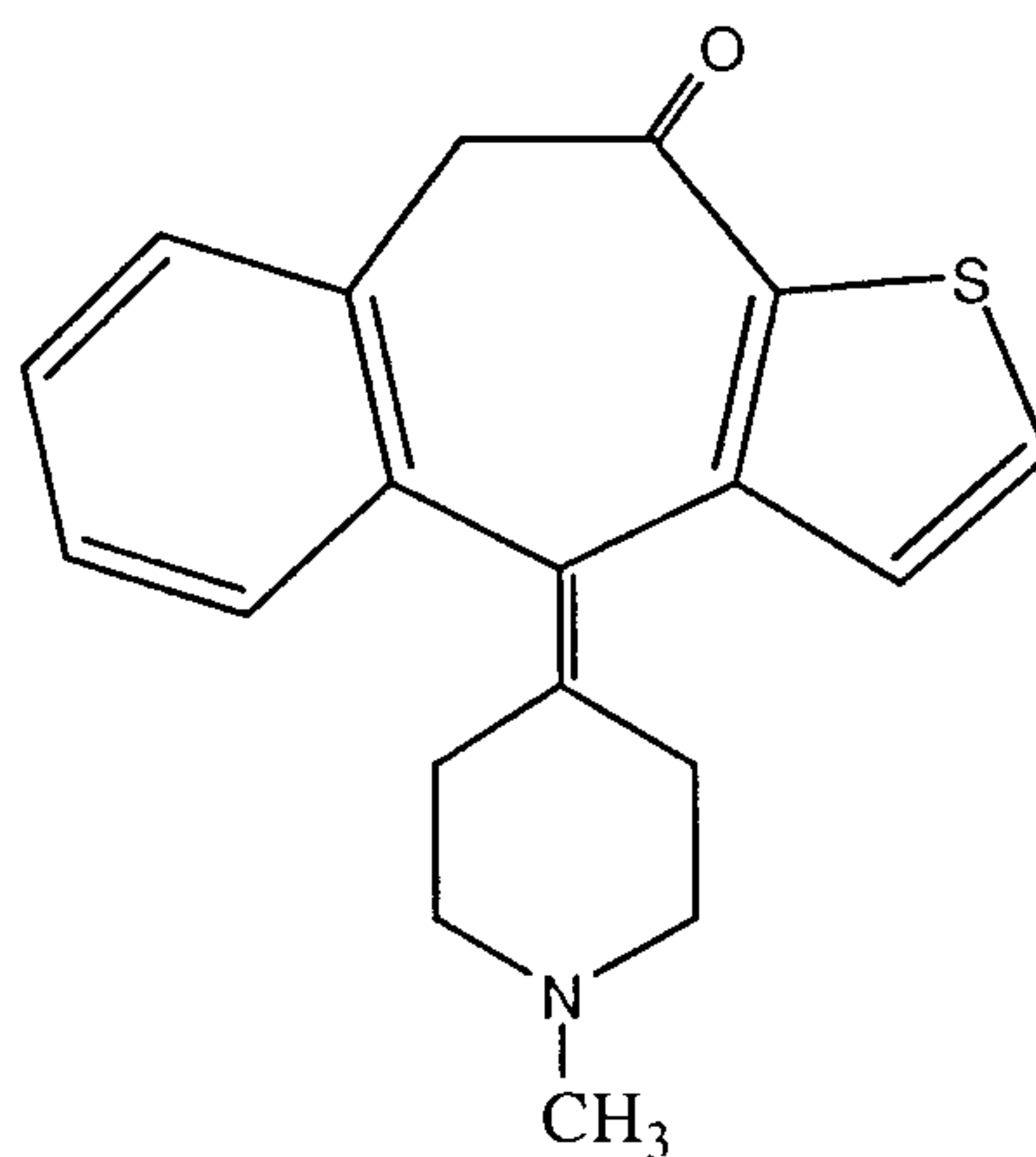
KETOTIFEN
