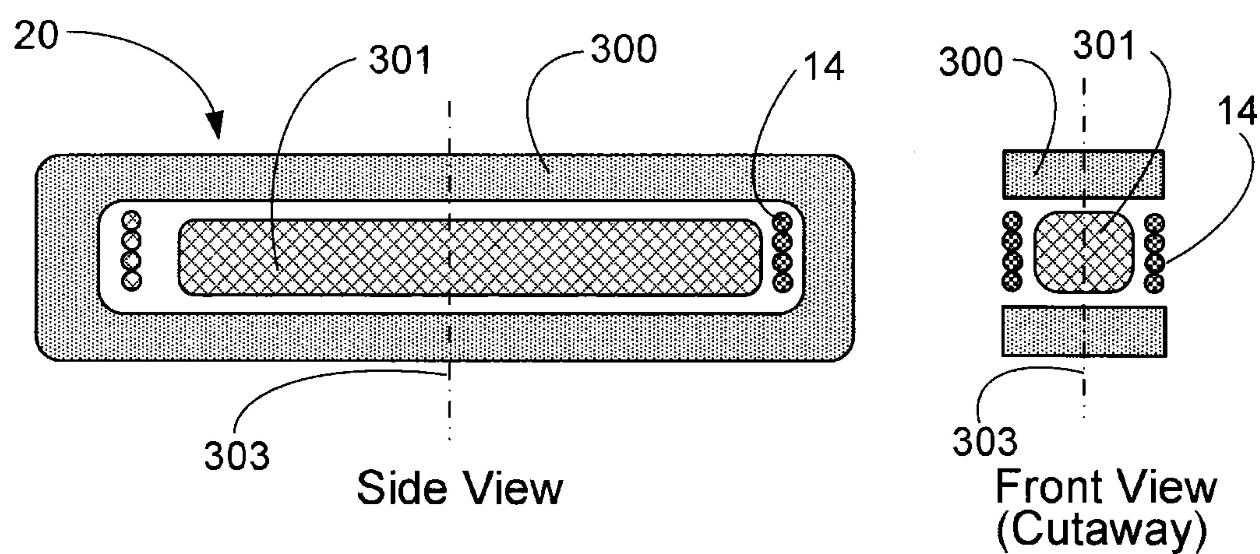
FIG. 3B
