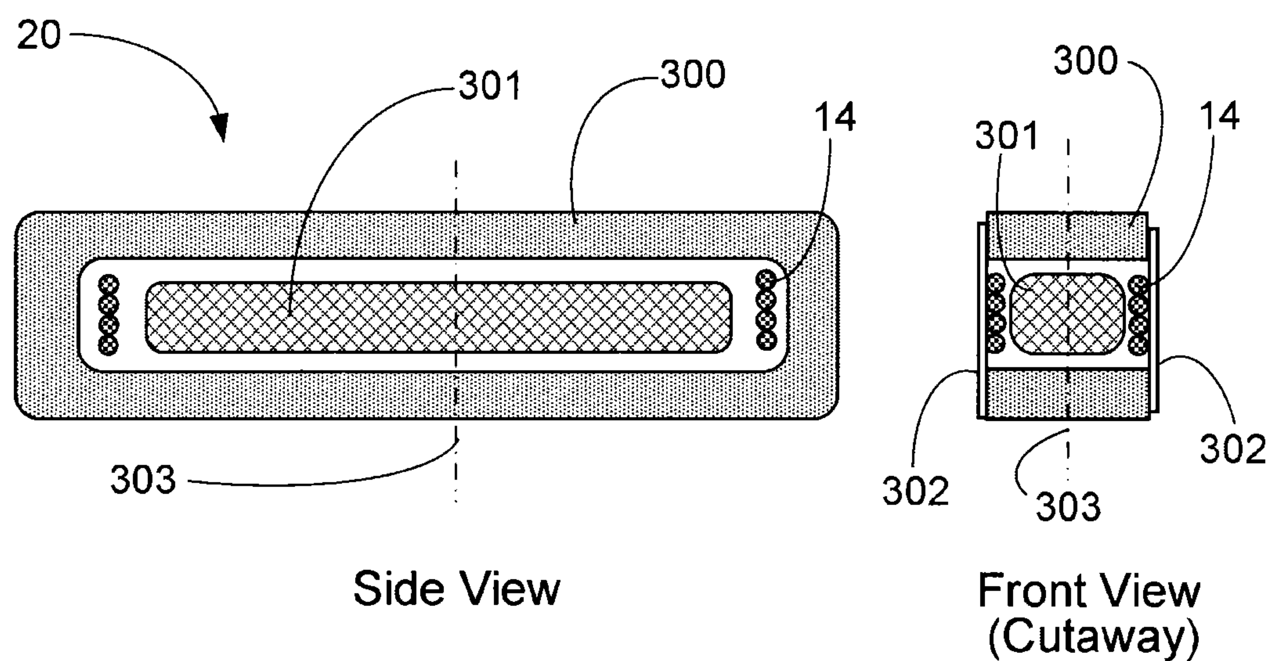
FIG. 3C
