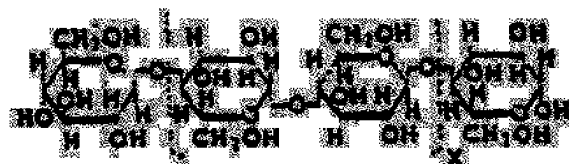
Молекула целюлози (Фиг. 2)
