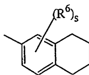
(a-43)
