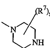
(a-51)
