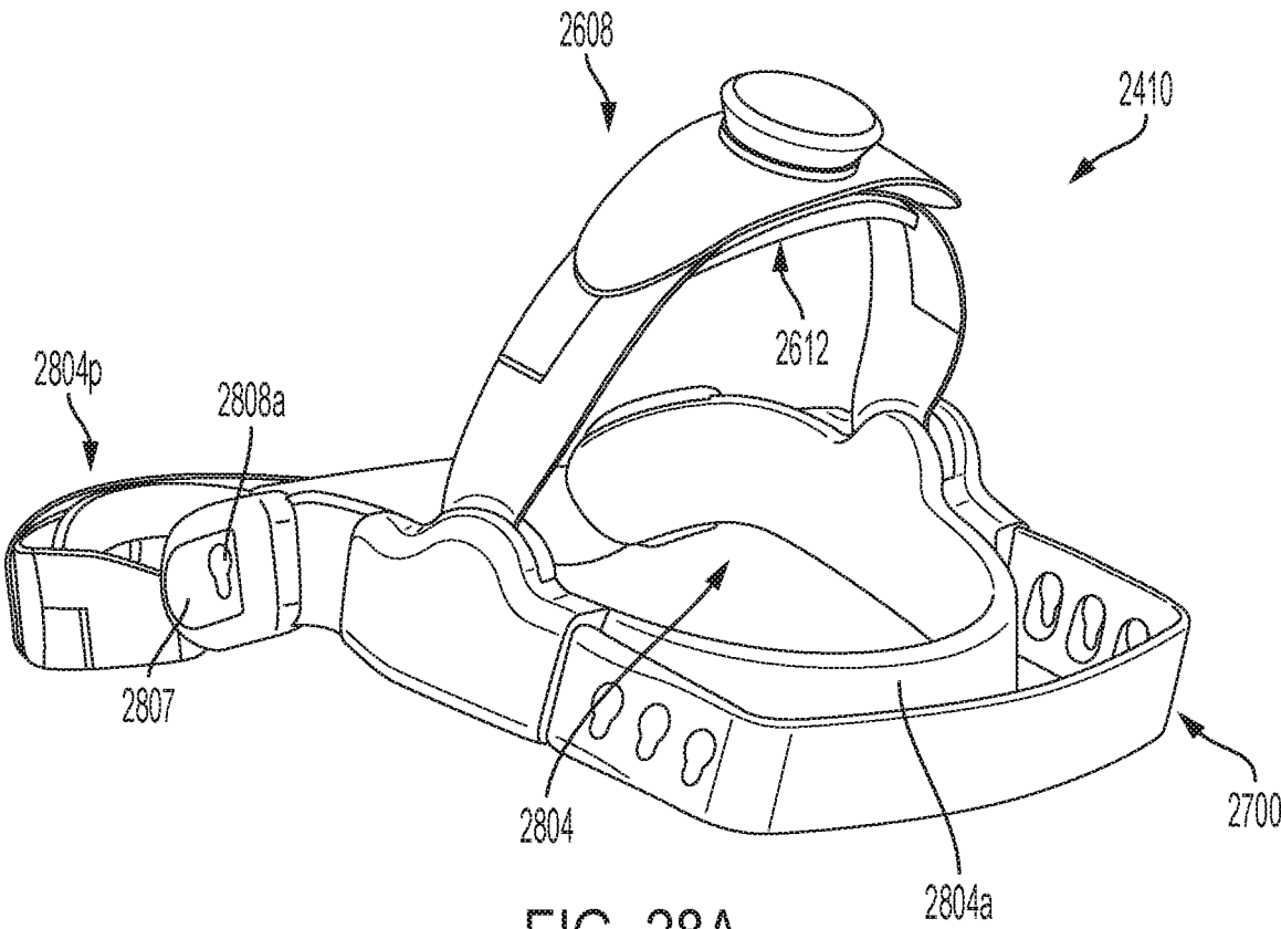
FIG. 28A
