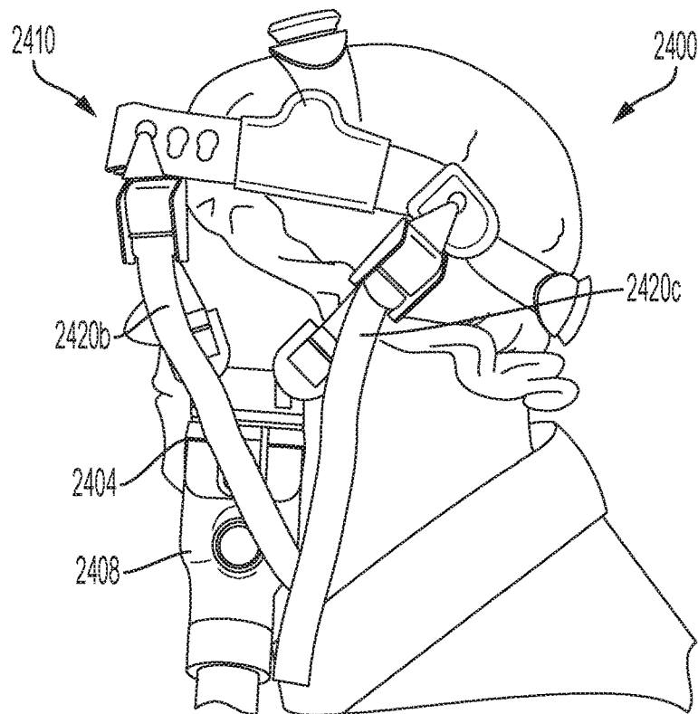
FIG. 24E
