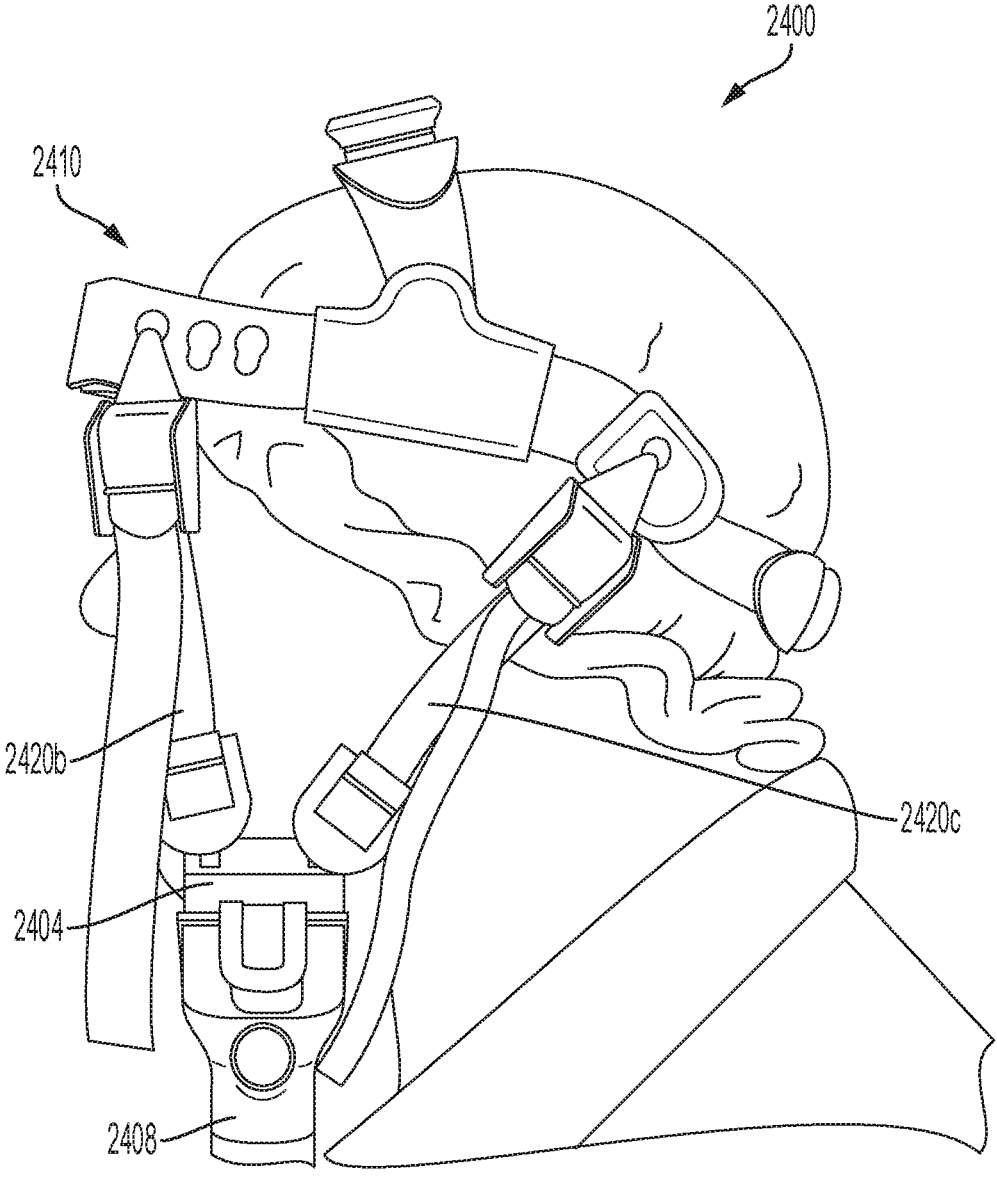
FIG. 24C
