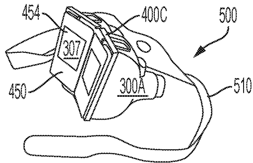
FIG. 18D
