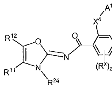
(IIId)
