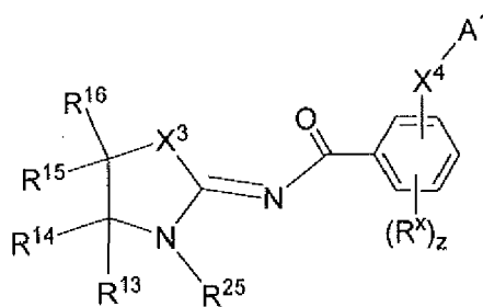
(Ie)
