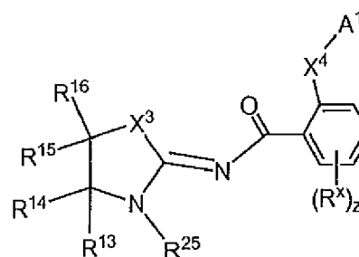
(IIe)
