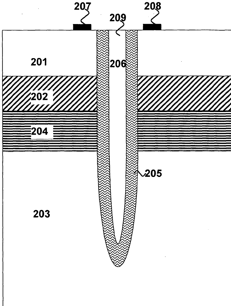
Fig. 2 : prior art
