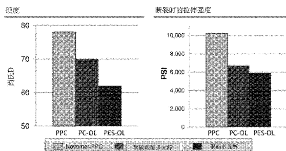
TPU中PPC的起始评价指示极高的硬度和拉伸强度
