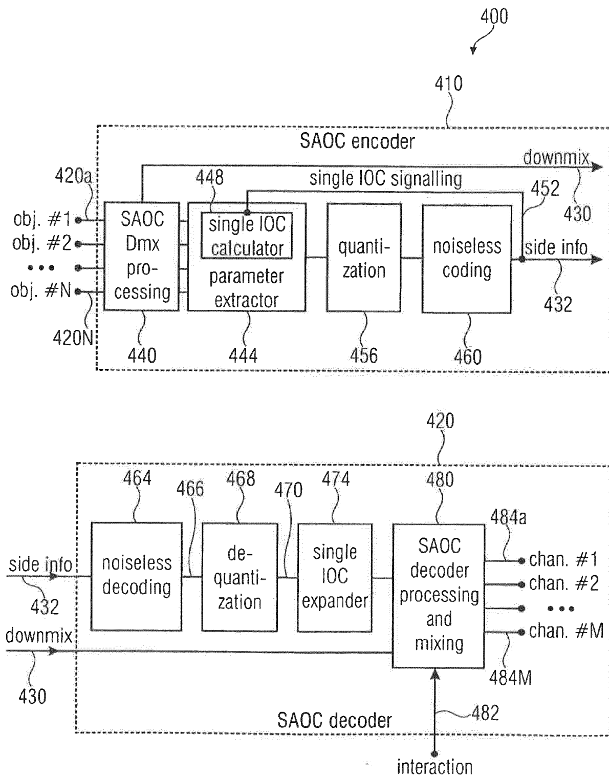
MPEG SAOC single IOC parameter calculation
