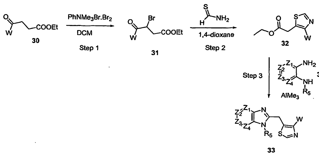
Scheme VI
