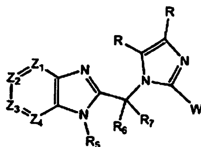
Formule A
