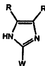
Formule B
